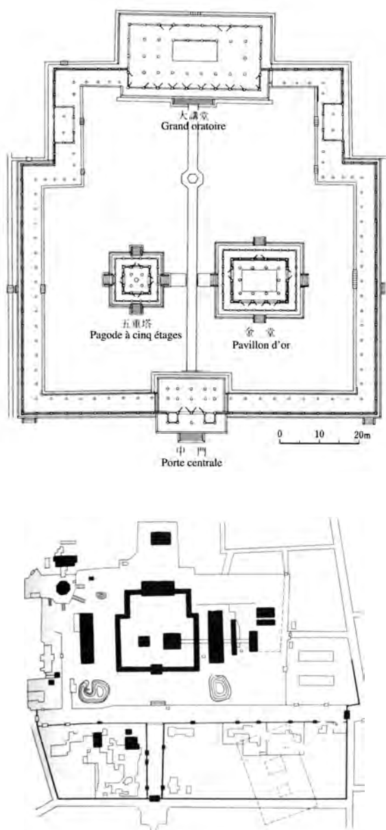
Fig. 5-6 - Monastère bouddhique, plans du Hōryūji (Nara). Bâtiments centraux dans la première enceinte (à gauche) et plan d'ensemble (à droite). Dessins adaptés de Nihon kenchiku-shi zushū ( Histoire illustrée de l'architecture japonaise ), éd. Nihon kenchiku gakkai.
