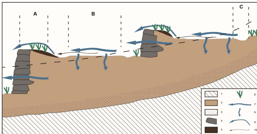
Figure 3. Schéma de fonctionnement des jessour
