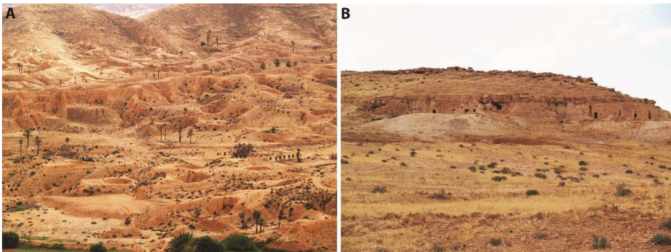
Figure 8. Habitations troglodytiques creusées dans la couverture loessique, entre Chemlali et Sidi Meta (A) et dans un banc de calcaire tendre à Ksar Hadada (B)
