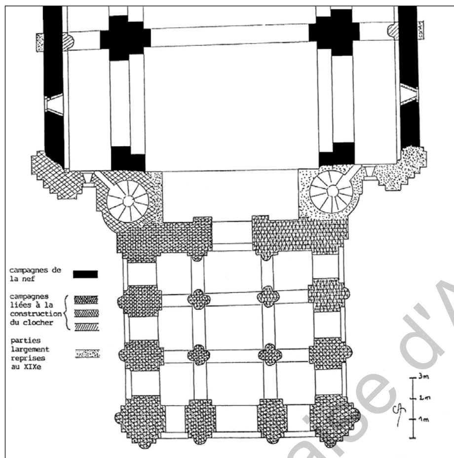
Fig. 11 - Lesteps (Charente), Saint-Pierre, clocher-porche et nef, plan au sol (relevés et tracés Cl. Andrault-Schmitt).
