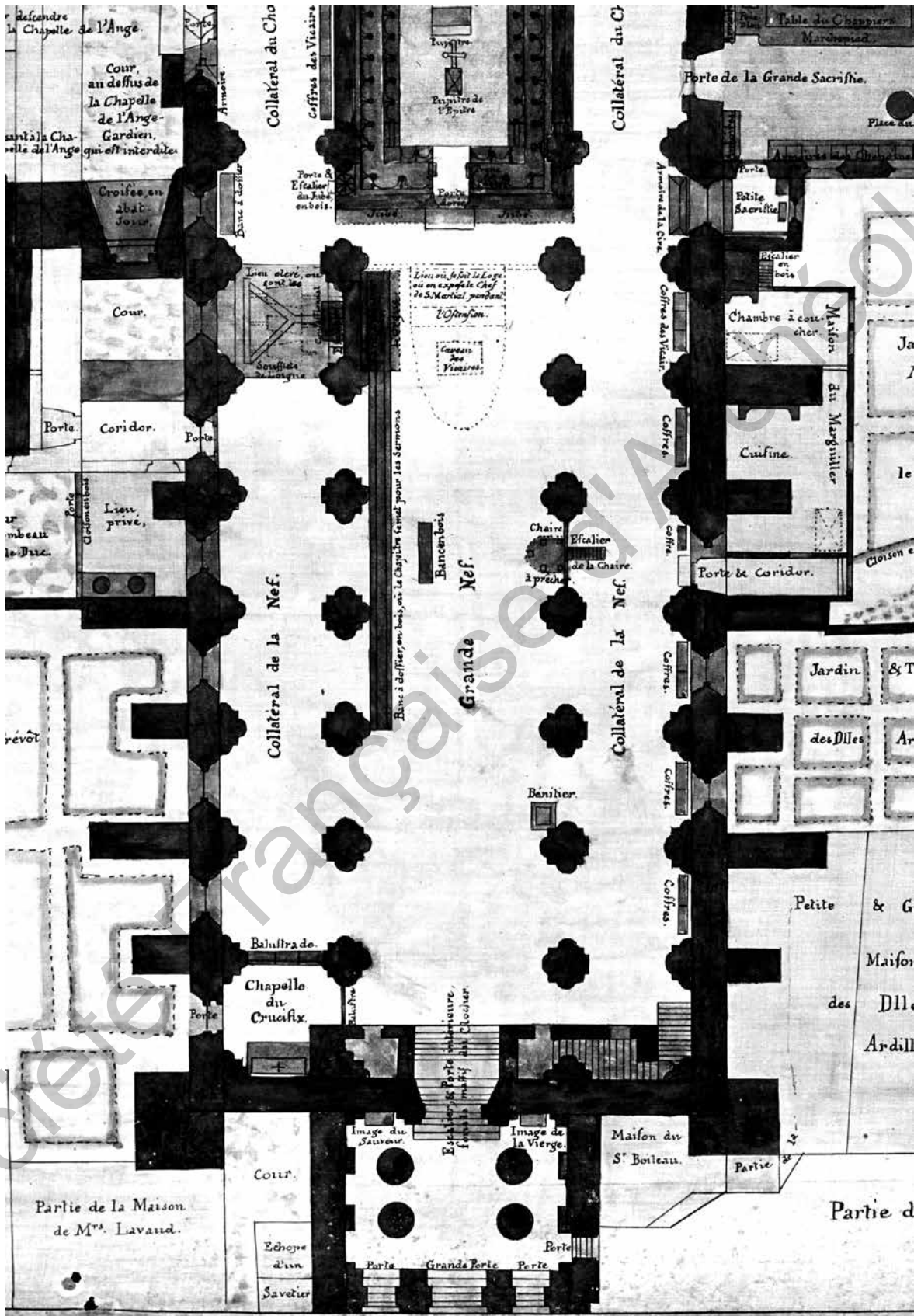
Fig. 1 - Limoges, Saint-Martial, plan de l'abbatiale du Sauveur par le chanoine Legros, partie occidentale (coll. part.).
