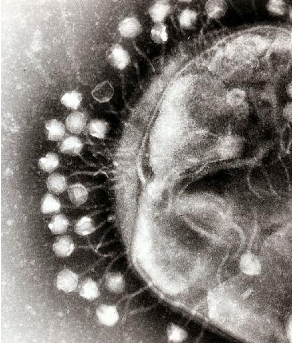
Microscopie électronique à transmission de virus bactériophages attachés par leurs fibres caudales à la membrane d'une bactérie. Crédit / Graham Beards
