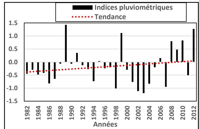
Fig. 2 : Indices pluviométriques à la station du Cap-Skirring (1982-2012)
