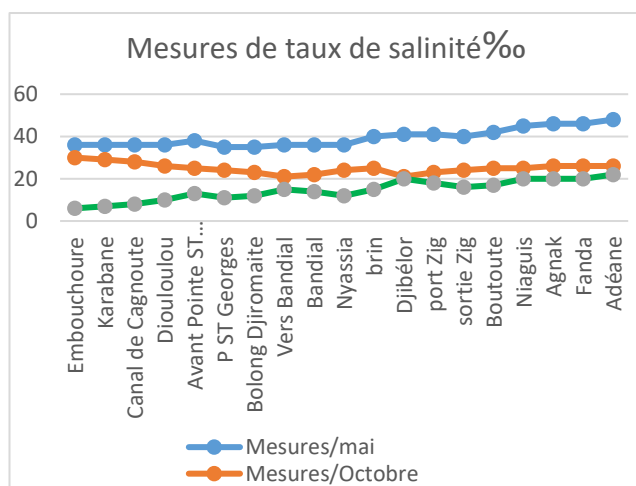
Fig. 5 : Variation de la salinité le long du chenal du fleuve Casamance (mai et octobre 2016)
