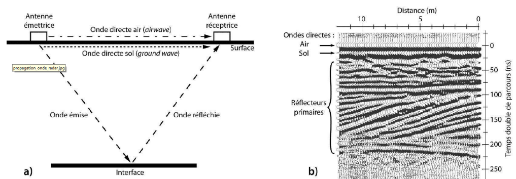
Fig. 4 Représentation schématique du principe de mesure de la diélectrique des sols et des résultats obtenus après traitement [d'après Neal 2004]
