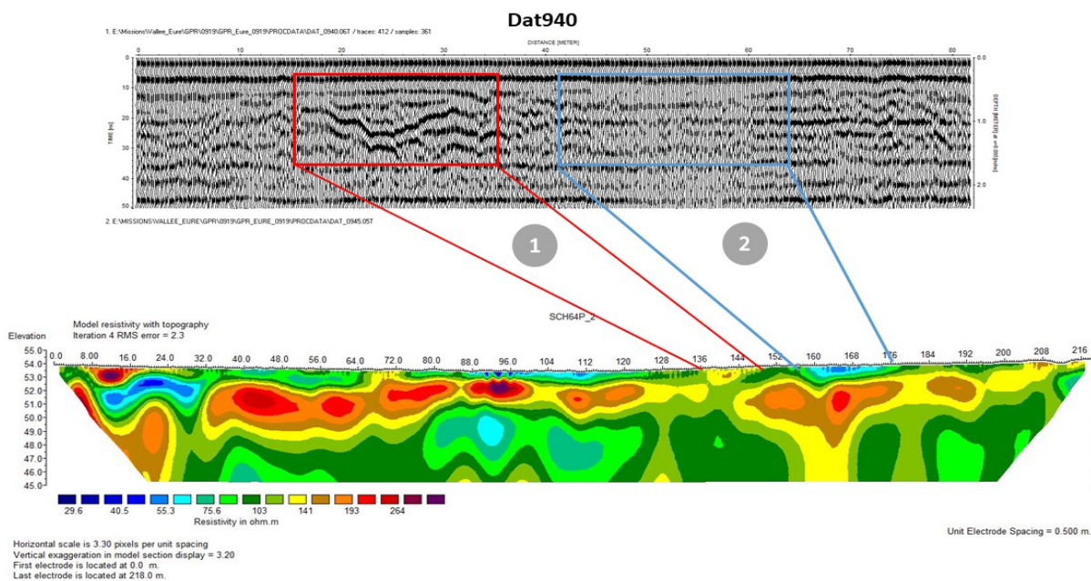
F g. 6 Profils géoradar et TRE réalisés dans le prolongement nord est du premier profil (fig. 4), à proximité immédiate du fanum (profils acquis le 11 septembre 2019) [traitement et réalisation Cl. Virmoux]
