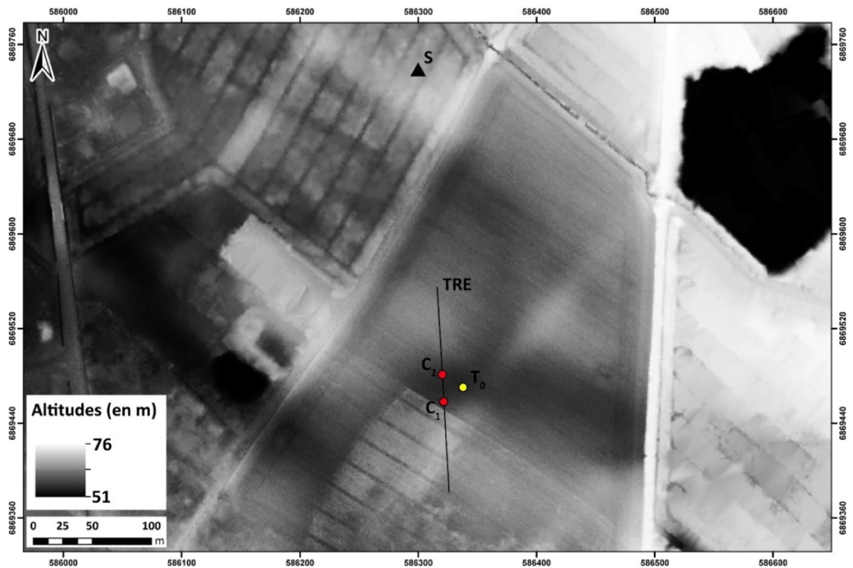
Fig. 3 Localisation du profil TRE perpendiculaire à l'axe du paléochenal et des deux carottages. Légende : S. Sanctuaire de Bellevue, TRE. Profil de résistivité électrique, T 0 . Sondage exploratoire à la tarière télescopique, C 1 et C 2 : carottages BEL I et II [Sources : RGE Alti 1 m et orthophotographie de l'IGN. Réalisation : T. Piau, 2019.
