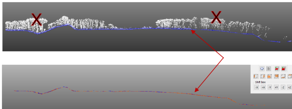
Fig. 4 Principe de calcul du MNT [I. Le Tellier, AirD'Eco Drones]
