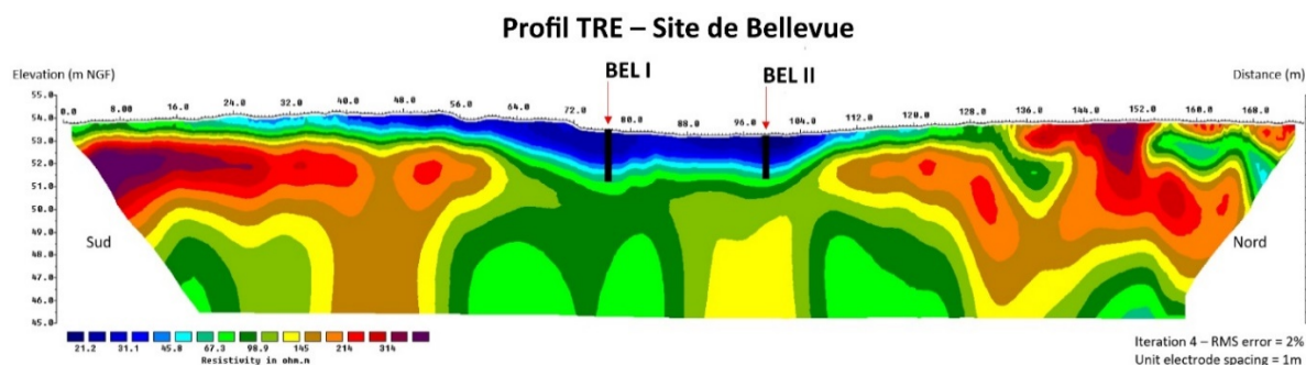
F g. 5 Profil de résistivité électrique perpendiculaire à l'axe du paléochenal de Bellevue (profil TRE acquis le 3 avril 2019). Les mesures de résistivité apparente forte en rouge renvoient à des faciès grossiers (grave à silex roulés) ; a contrario, les mesures de résistivité apparente faible (en bleu et vert) renvoient à des faciès sédimentaires plus fins (argiles et limons) [traitement et réalisation Cl. Vermoux]
