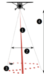
F g. 2 Rappel théorique sur les principes du LiDAR : 1. longueur d'onde : 1550 nm/ 1064 nm (topographie) ; 532 nm (bathymétrie) ; 355nm (atmosphérique) ; 2. angle du scanner / fauchée ; 3. vitesse de balayage ; 4. altitude de vol [1. Le Tellier, AirD'Eco Drones]
