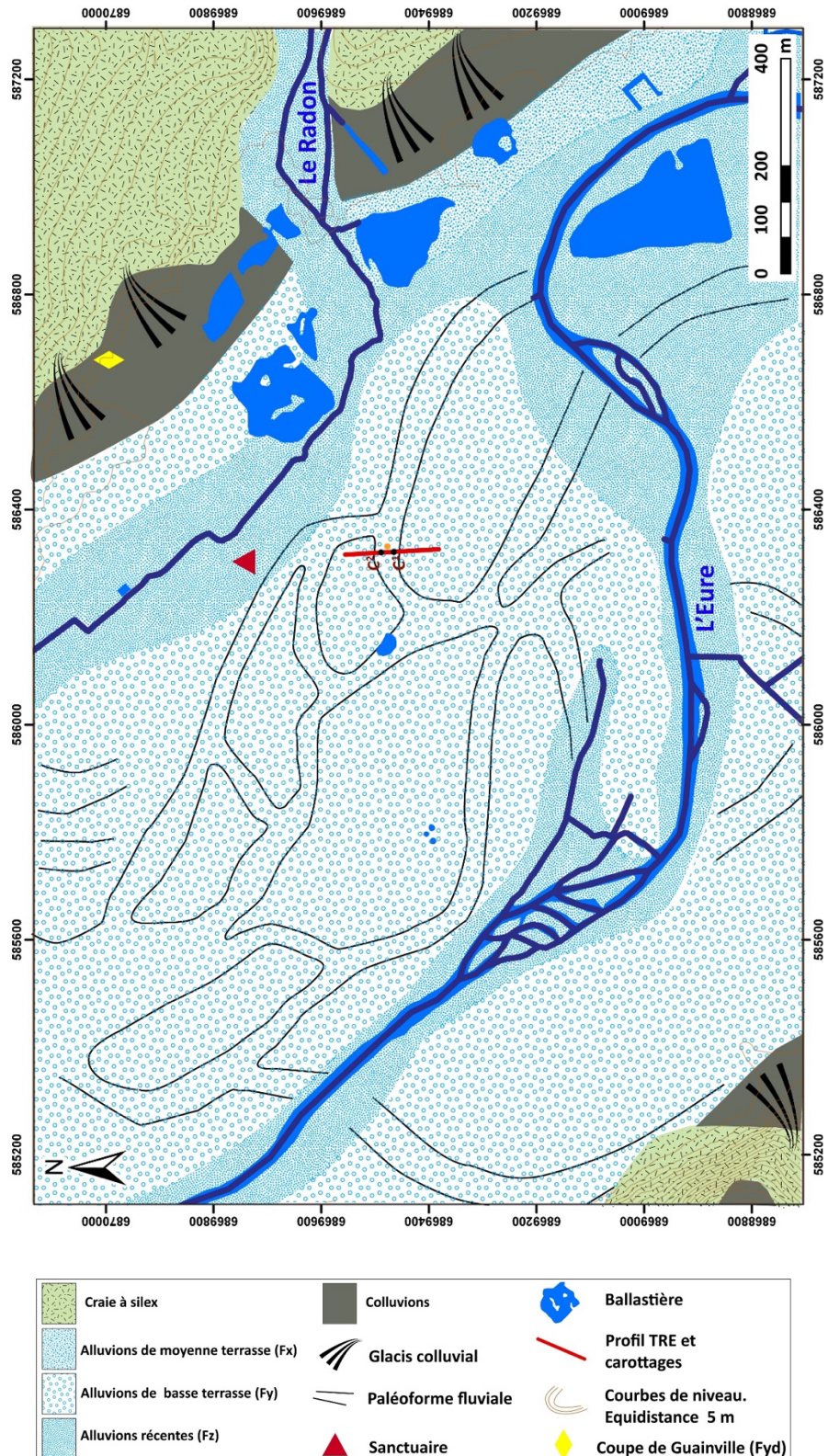
F g. 2 Croquis géomorphologique interprétatif du site de Bellevue [Sources : RGE Alti 1 m et BD Carthage. DAO Th. Piau, 2019]
