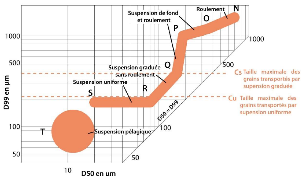
F g. 3 Image CM de Passega [d'après Passega 1964, adapté par Beauchamp 2019]
