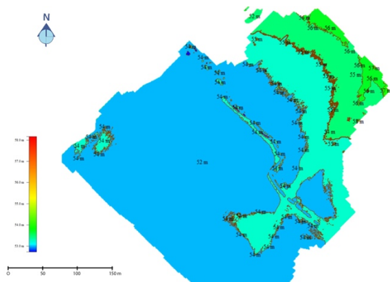
Fig. 9 Classification des points et traitement par courbes de niveau à 1 m et 0,5 m [source : I. Le Tellier, AirD'Eco Drones]
