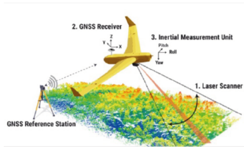
F g. 2 Rappel théorique sur les principes du LiDAR : 1. longueur d'onde : 1550 nm/ 1064 nm (topographie) ; 532 nm (bathymétrie) ; 355nm (atmosphérique) ; 2. angle du scanner / fauchée ; 3. vitesse de balayage ; 4. altitude de vol [1. Le Tellier, AirD'Eco Drones]
