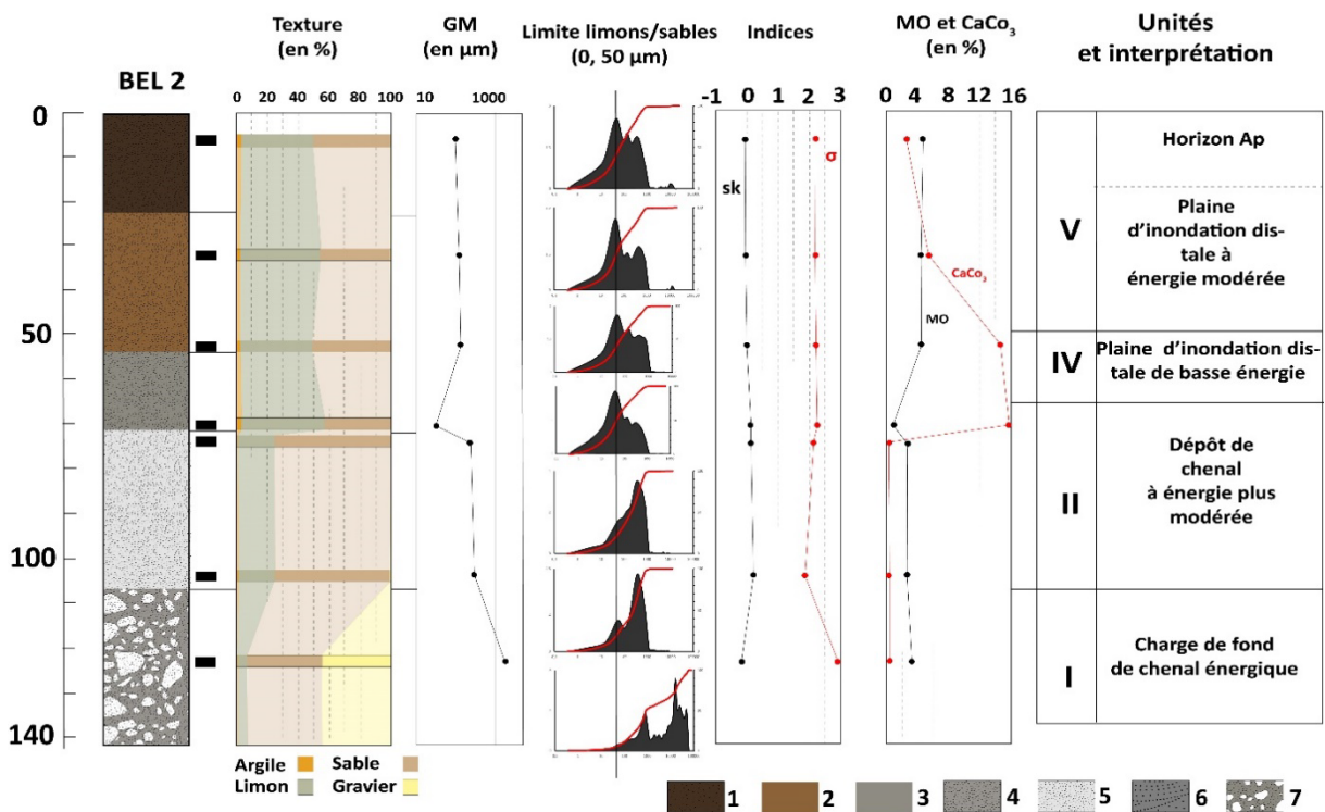
F g. 5 Analyses sédimentologiques des logs BEL I et II. 1. Horizon Ap cultivé ; 2. Limons sableux bruns ; 3 et 4. Limon sableux gris à traits rédoxiques (horizon g) ; 5. Sables limoneux à intercalation de sables ; 6. Sables graveleux [d'après Piau 2019]
