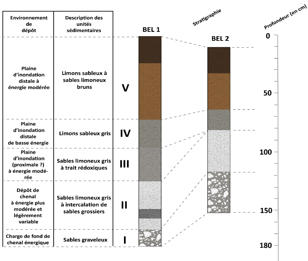
F g.4 Interprétation en termes de milieux de sédimentation des unités sédimentaires décrites à partir des sondages BEL I et BEL II réalisés dans le remblaiement du paléochenal de Bellevue [d’après Piau 2019]
