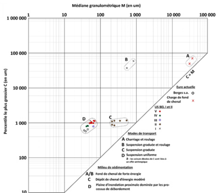
F g. 6 Image CM/Passéga des unités sédimentaires du paléochenal de Bellevue : interprétation en termes de modes de transport et de milieux de sédimentation [d'après Piau 2019]
