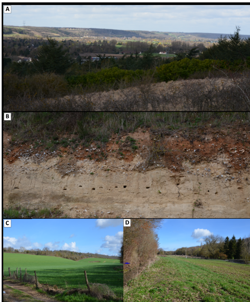
26 A Vue en direction du nord-est de la vallée de l'Eure depuis le plateau en rive droite en aval de la Chaussée-d'Ivry. De part et d'autre de la vallée de l'Eure, la surface de ce plateau correspond pro-parte à une surface substructurale éocène. Ce panorama permet d'observer, au second plan, le versant crayeux de la rive gauche de l'Eure réglé par le sapement fluvial et les processus périglaciaires quaternaires. B Terrasse alluviale de Guainville. Par analogie avec d'autres séquences alluviales décrites par Y. Dewolf (1970) dans la vallée de l'Eure à la même altitude (Bueil, Chaudon), cette séquence est probablement d'âge saalien. Elle est composée d'une alternance de sables fins à grossiers orangés plus ou moins limoneux ou argileux contenant des intercalations de lits subhorizontaux à galets de silex anguleux à sub-émoussés. Des dépôts tufacés sont identifiés dans le comblement d'un paléochenal dans la partie médiane de l'affleurement. La partie sommitale de la coupe est constituée d'un niveau à cailloutis de silex emballés dans une matrice argilo-sableuse ferruginisée (paléosol éémien ?) affectée par des figures de cryoturbation, fentes de gel et coins de glace, à rapporter au Weichsélien. Ce paléosol est recouvert de limons éoliens mêlés à des colluvions weichséliennes en provenance du versant. C Basse vallée du Radon. Noter le faible remblaiement alluvial, le versant se raccordant directement au fond de vallée. D Glacis colluvial identifié dans la moyenne vallée du Radon. Noter également le fossé de drainage agricole à l'extrémité gauche de la photographie, interrompant le glacis colluvial [© Th. Piau et Fr. Bétard 2019]
