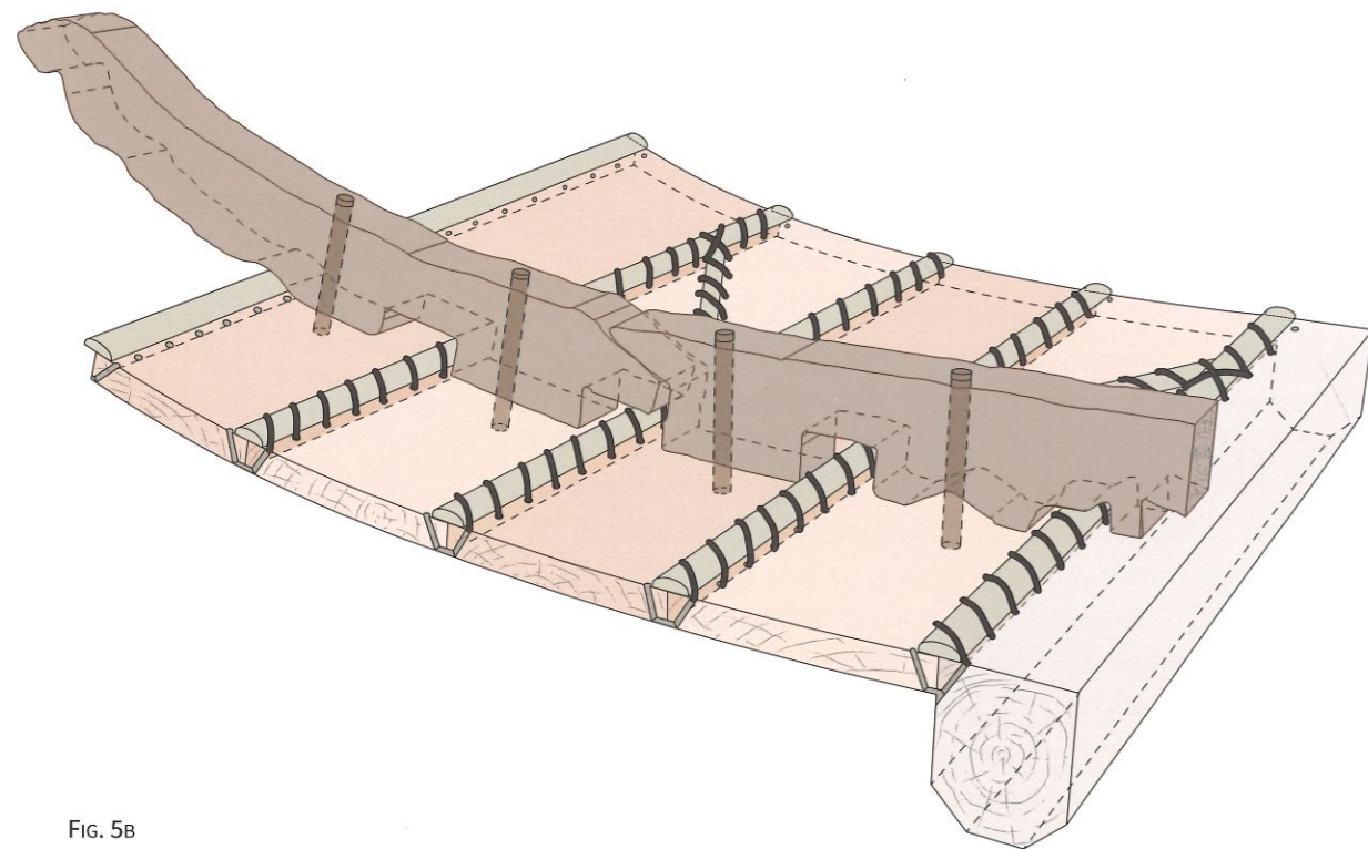
FIG. 5B. Sistema di giunzione della chiglia, dei corsi del fasciame e delle ordinate di una tipica barca cucita d'epoca romana utilizzata in Istria e Dalmazia settentrionale. Diversamente dalla tradizione greca, i corsi del fasciame sono collegati da un sistema di cuciture più semplice che prevede un solo passaggio di una treccia vegetale nei canali che attraversano le tavole del fasciame. Il cuscinetto ammortizzatore è costituito da fibre vegetali e le trecce sono bloccate da spinotti. Le ordinate, a sezione rettangolare, sono munite dei tipici incassi alla base e sono collegate al fasciame mediante cavicchi lignei (disegno P. Poveda, Aix-Marseille Université, CNRS, CCJ).
