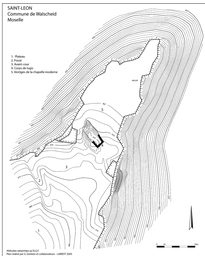
Fig. 2. Château de Walscheid. Plan G. Giuliano, 2001.
