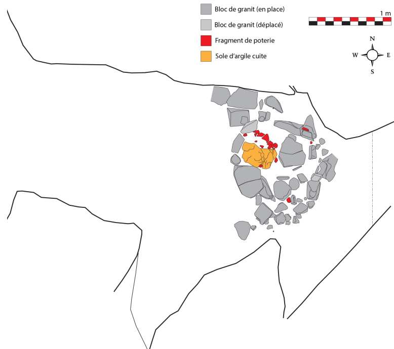
Fig.4. Tiresa, plan de l'abri 1 (travaux P. Nebbia, relevé P. Tramoni, DAO K. Peche-Quilichini). Tiresa, planimetry of shelter n.1 (excavations P. Nebbia, drawing P. Tramoni, edrawing K. Peche-Quilichini).
