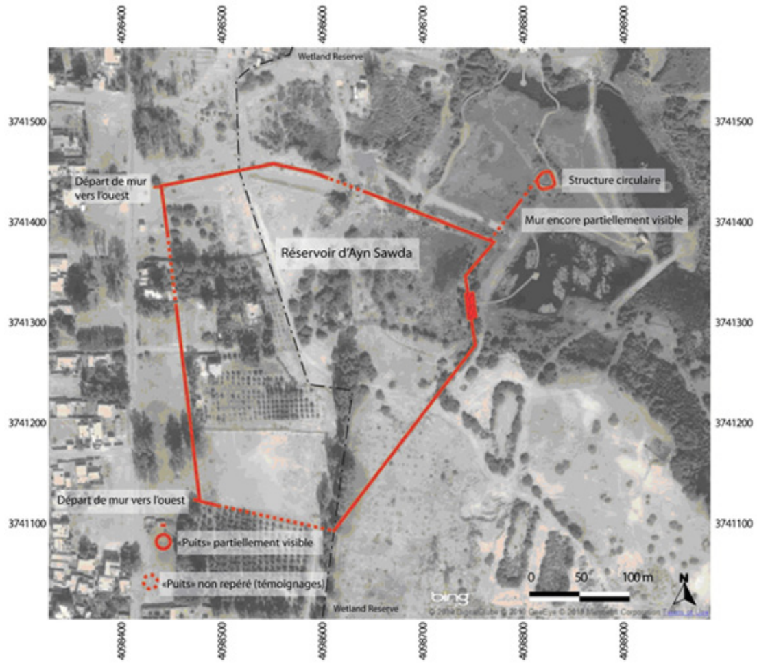
Fig. 16. Image satellitaire du réservoir d'Ayn Sawda et indication des structures présentes sur le site (L. Abu-Azizeh).
