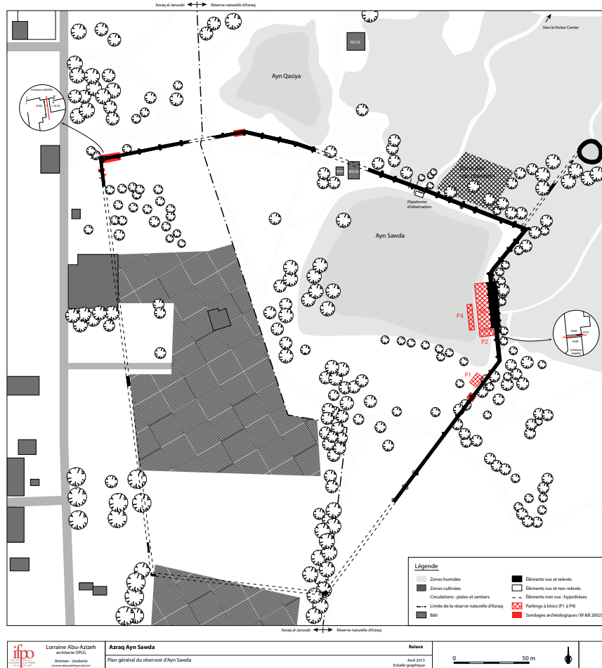
Fig. 20. Nouveau plan topographique (site et contextes) (L. Abu-Azizeh).
