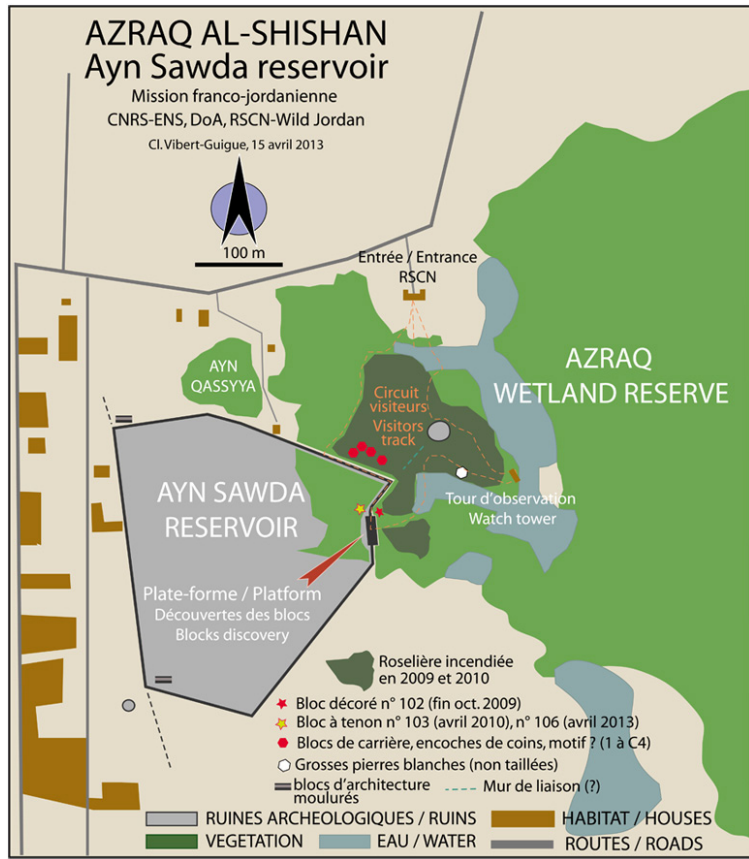
Fig. 1. Plan schématique évolutif (Cl. Vibert-Guigue).
