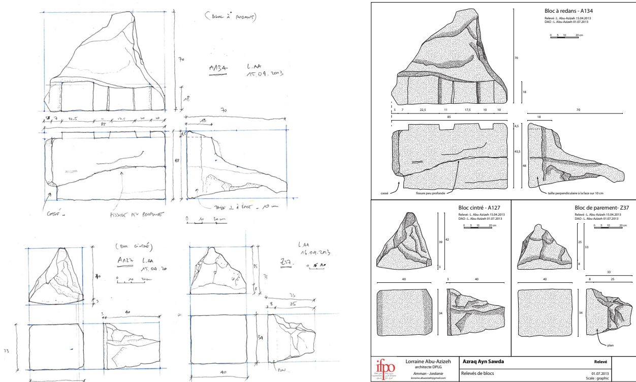
Fig. 22. Exemple d'étude de bloc : relevés de terrain et mise au net par L. Abu-Azizeh.
