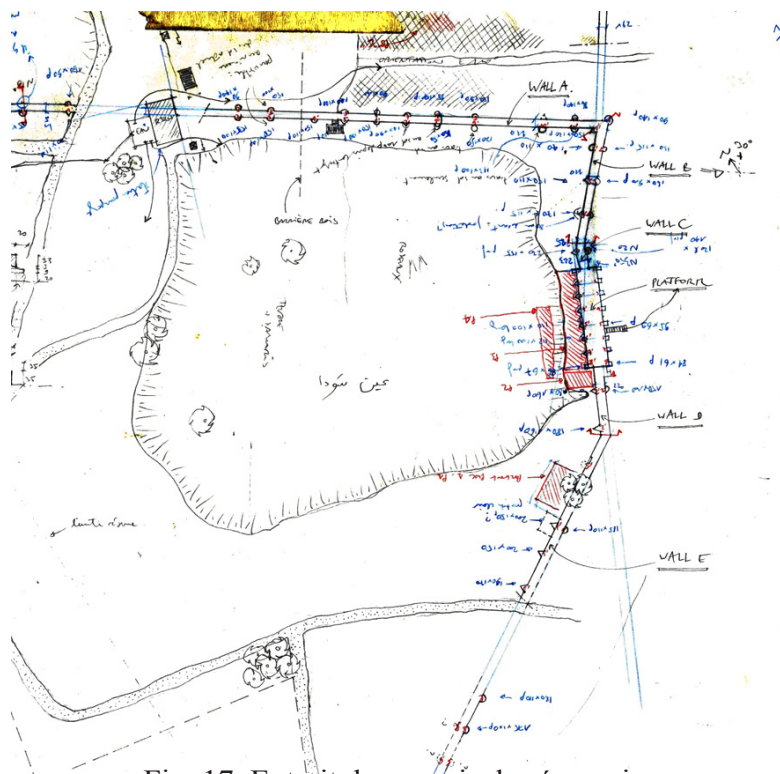
Fig. 17. Extrait du croquis du réservoir (L. Abu-Azizeh).
