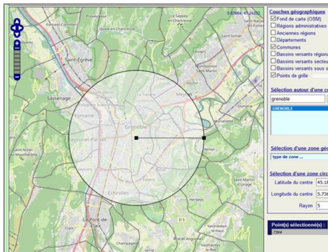
Figure 2. Aire de 5 km autour de Grenoble correspondant au point de grille SAFRAN (point 7394) ayant servi à calculer les données T_n et T_x , d'altitude moyenne 284 mètres, pour le climat futur (2006-2100) ; d'après un extrait du portail Drias. Area of 5 km around Grenoble corresponding to the SAFRAN grid point (point 7394) used to calculate the T_n and T_x data for future climate (2006-2100), with an average altitude of 284 meters; from Drias portal.
