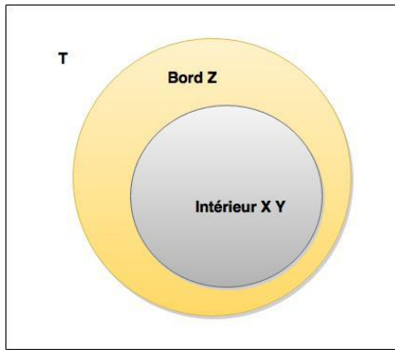
Figure 1 : Topologie de la partie (x, y, z)
