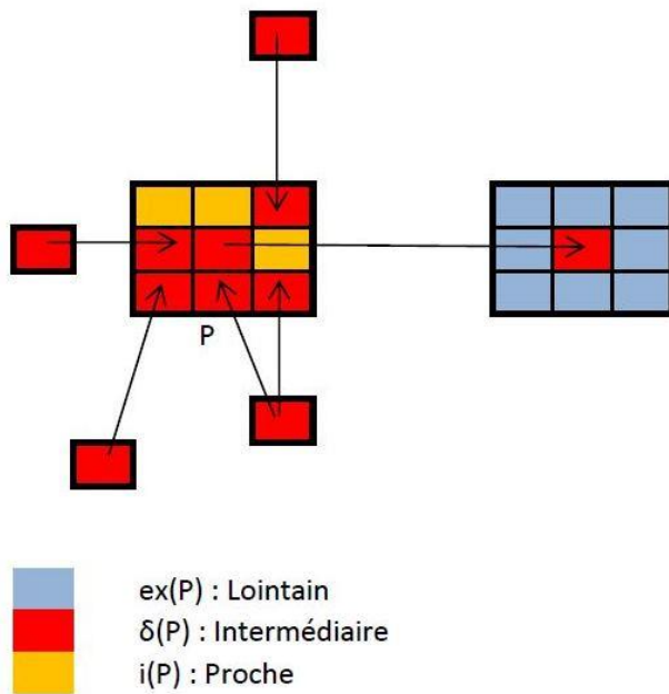
Figure 4 : Prétopologie urbaine du domicile travail
