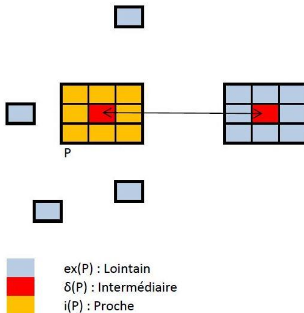
Figure 3 : Prétopologie urbaine du navetteur interurbain
