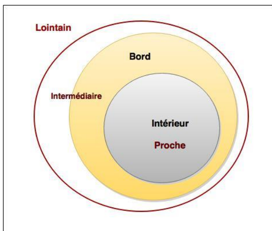
Figure 2 : Du proche au lointain
