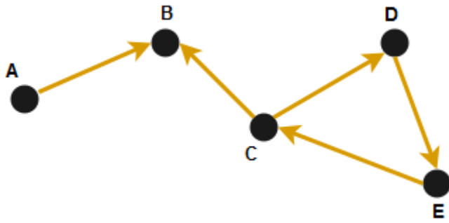
Figure. 9 Un réseau ..... non connexe.
