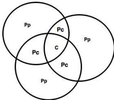
Figure 6 : Communauté de parties.
