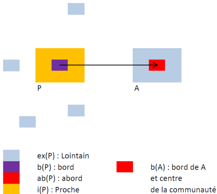
Figure 7 : Exemple de communauté.
