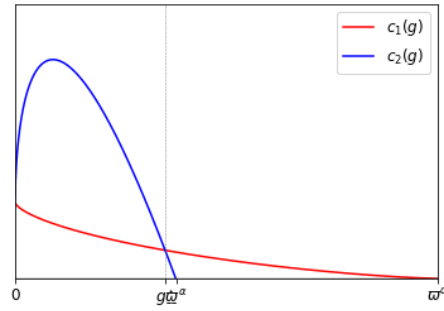
(d) Unique steady state with c'_2(g^*) < c'_1(g^*)
