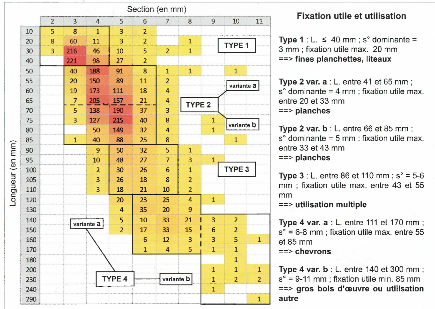
Fig. 5 : Mise en évidence des différents types de clou à partir des longueurs et des sections, et une description synthétique par type (DAO : V. TAILLANDIER et F. BLONDEL).
