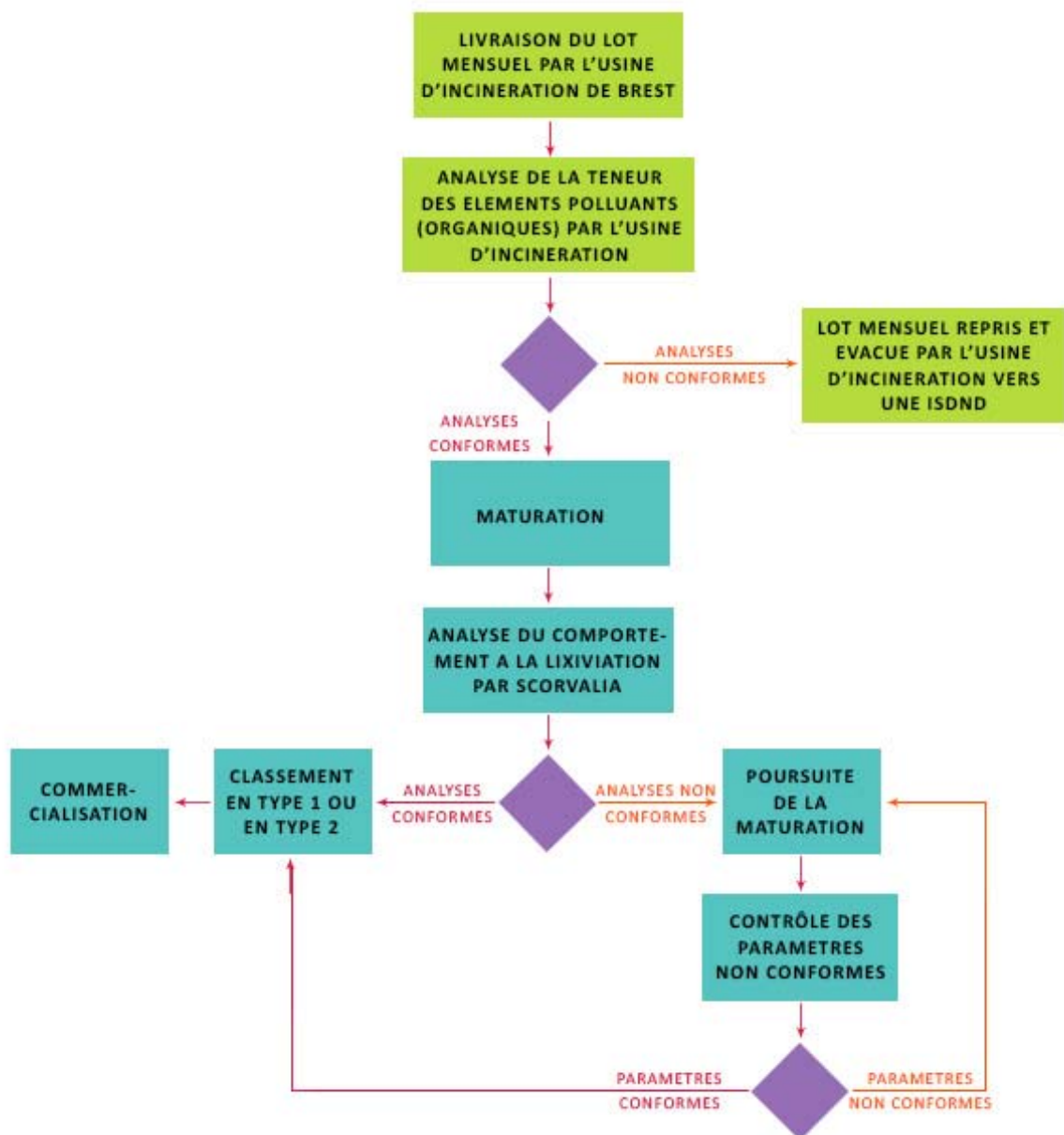
Circuit du mâchefier brut au Scorgrave ® (source : Symeed29, Finistère)
