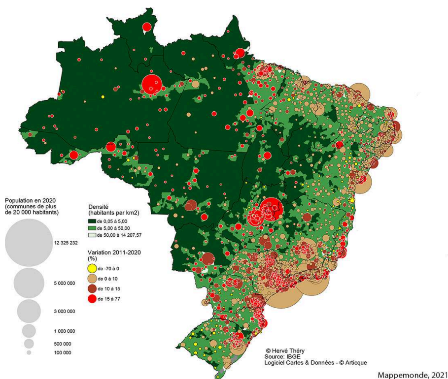
Figure 11. Population, densité démographique et évolution de la population communale du Brésil entre 2011 et 2020
