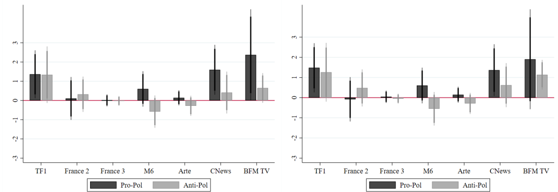
(c) \ln(Sub_{ct-1})
