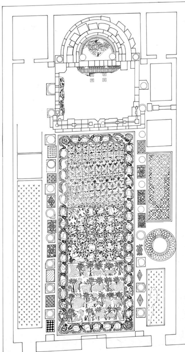
Fig. 10. Pianta della chiesa del Khadir di Madaba (Piano U. Lux, C. Florimont, E. Alliaia, 1966-1992) (Bikai 1996, p. 29). Le tracce del supporto del ciborium non sono rilevate e gli incastri, pur se visibili nello stilobate del presbiterio, non sono tutti indicati (vedi fig. 11).
