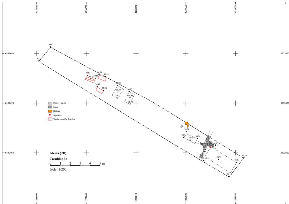
Fig. 1 – Plan général de la tranchée de J. Jehasse et relevé pierre à pierre des maçonneries
