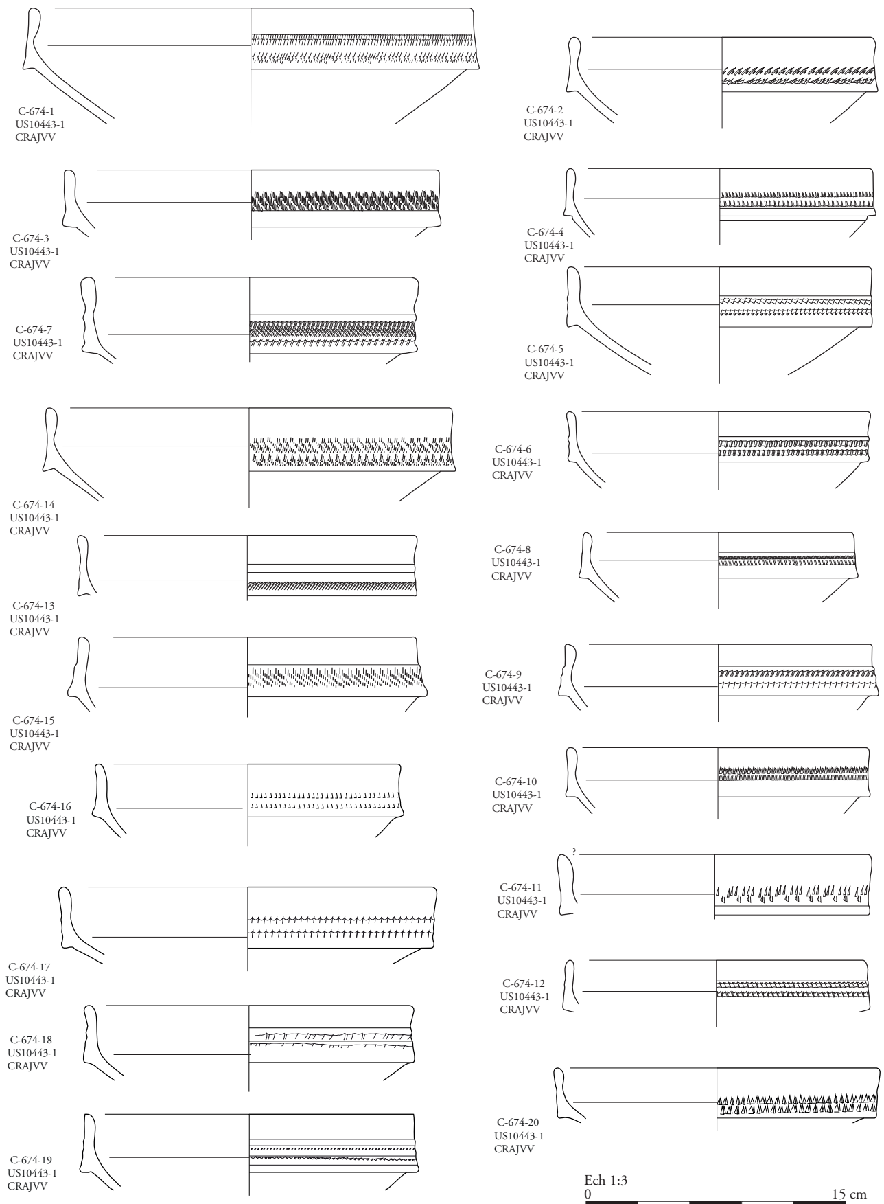
Pl. 173 : Site 1c. Mobilier céramique de l'épan dage F10443. Dessins : D. Champeaux ; DAO : D. Champeaux, A. Gilles ; éch. 1/3.
