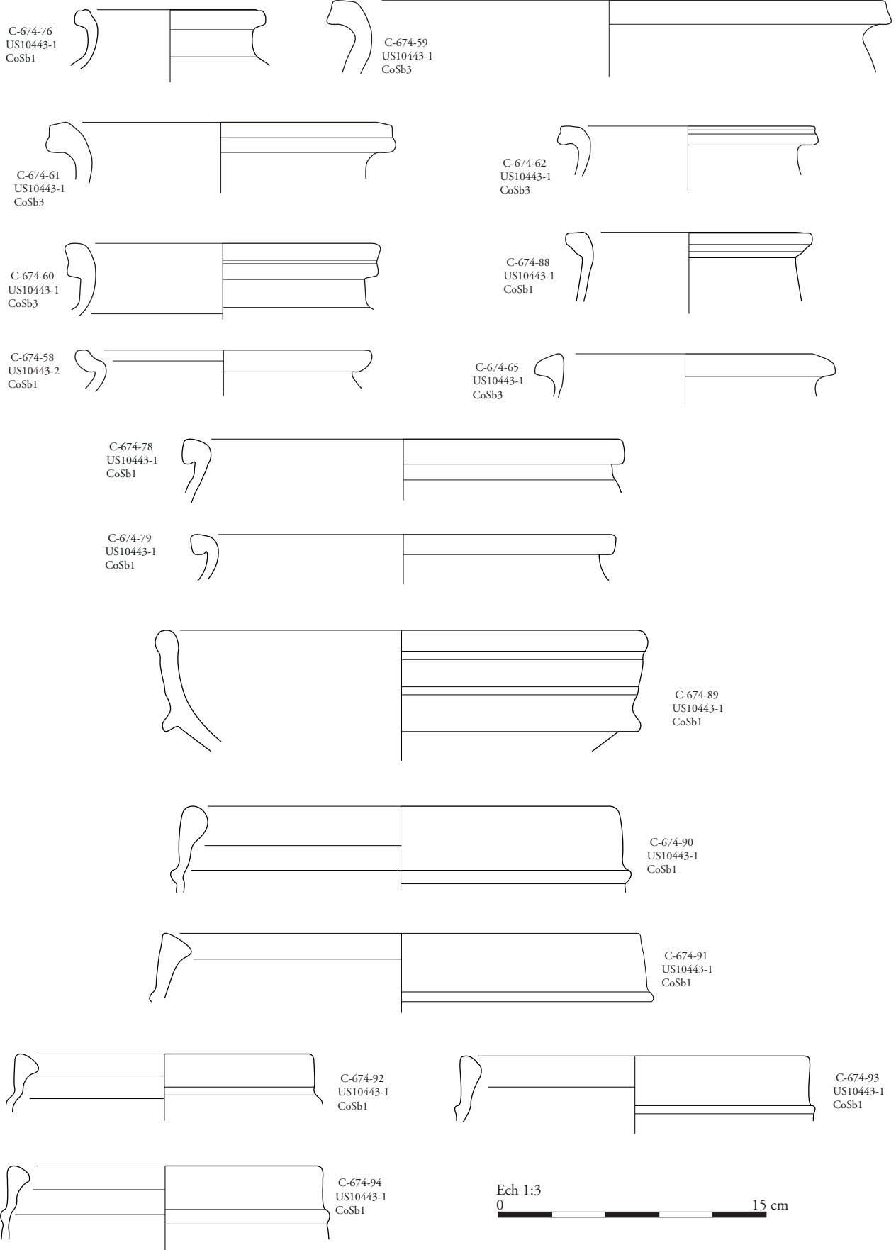
Pl. 177 : Site 1c. Mobilier céramique de l'épan dage F10443. Dessins : D. Champeaux; DAO : D. Champeaux, A. Gilles; éch. 1/3.
