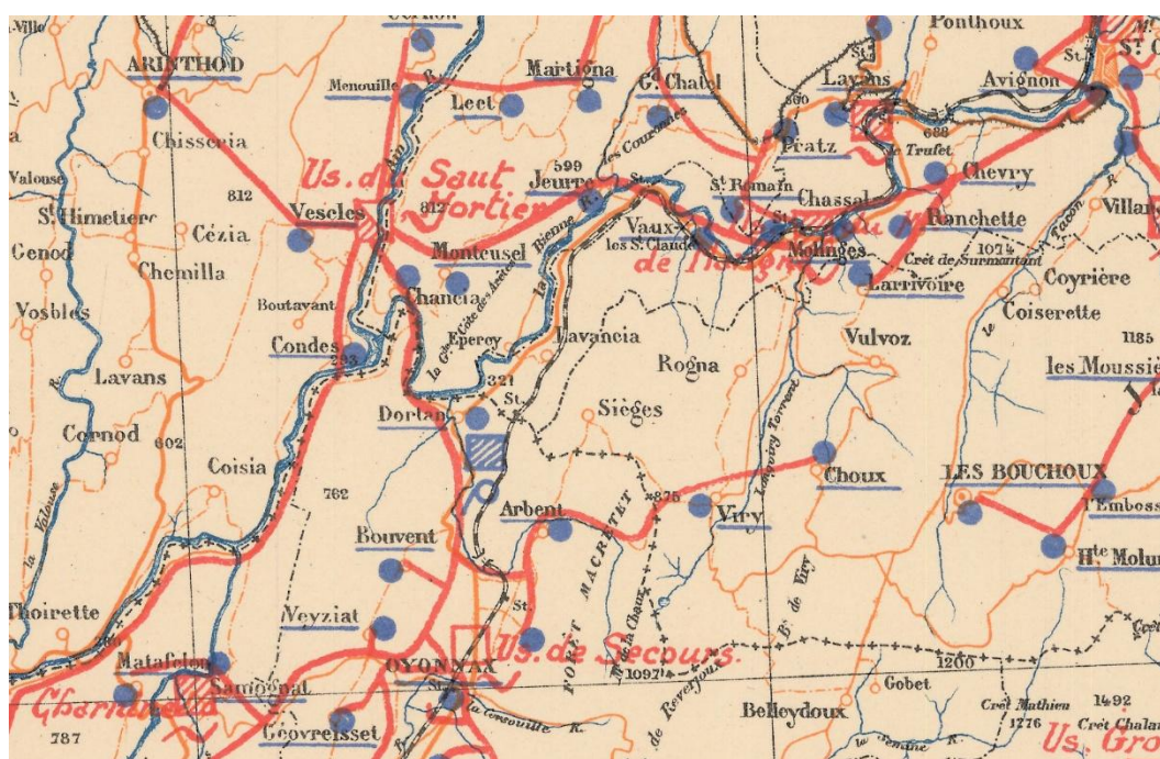
F1880_06/b. Distribution d'énergie électrique au 1:200 000, extrait exemplaire Extrait de la feuille n° 48, Anancy , Paris, Ministère des Travaux publics et des transports, s.d. [1918].
