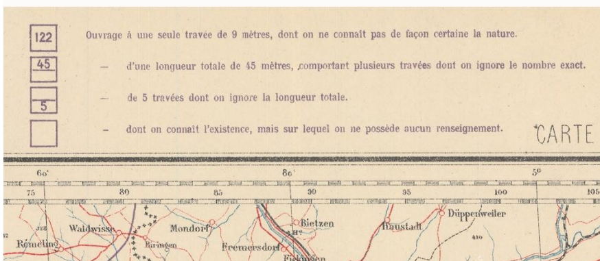
F1880_07/b. Capacité des ponts au 1:200 000, légende Huit signes conventionnels, complétés par des valeurs chiffrées, qualifient chaque ouvrage par son mode et son matériau de construction, par le nombre de ses travées et sa longueur. – Extrait de la feuille n° 18, Metz, Paris, Service géographique de l'armée, s.d. [ca. 1920].
