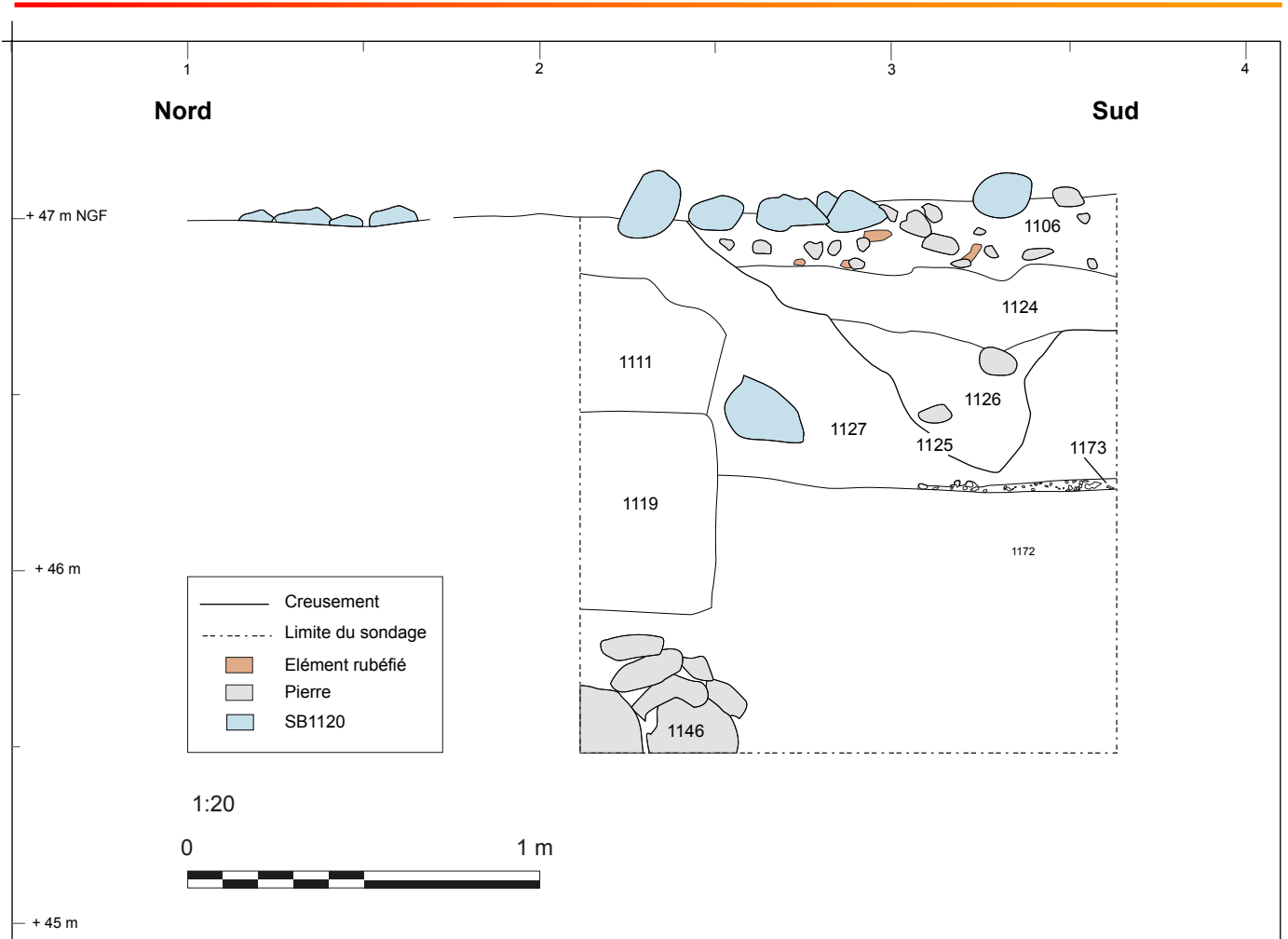
Fig. 13 : Relevé de la coupe 1S4 montrant face est du sondage 6 (d'après le relevé photogrammétrique de S. Sanz-Laliberté ; DAO : A. Vacheret)
