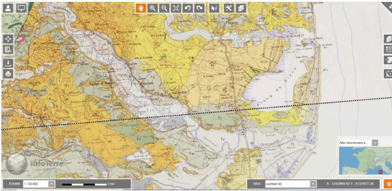
Fig. 2 : Carte géologique correspondante à la zone couverte par la fig. 1 (extraits des cartes géologiques n°1115 Pietra-di-Verde et n°1119 Ghisonaccia au 1/50.000e- assemblage des cartes Visualiseur InfoTerre).
