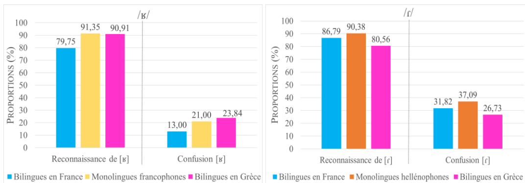
FIGURE 2 - Pourcentages généraux de reconnaissance et de confusions de /ʁ/ (à gauche) et /r/ (à droite)
