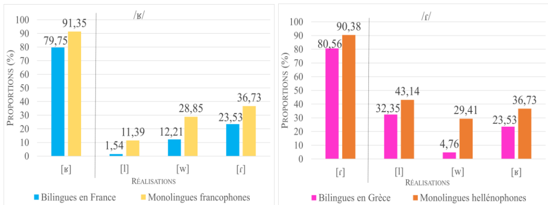
FIGURE 1 - Pourcentages de reconnaissance et détail des confusions de /ʁ/ (à gauche) et /r/ (à droite)
