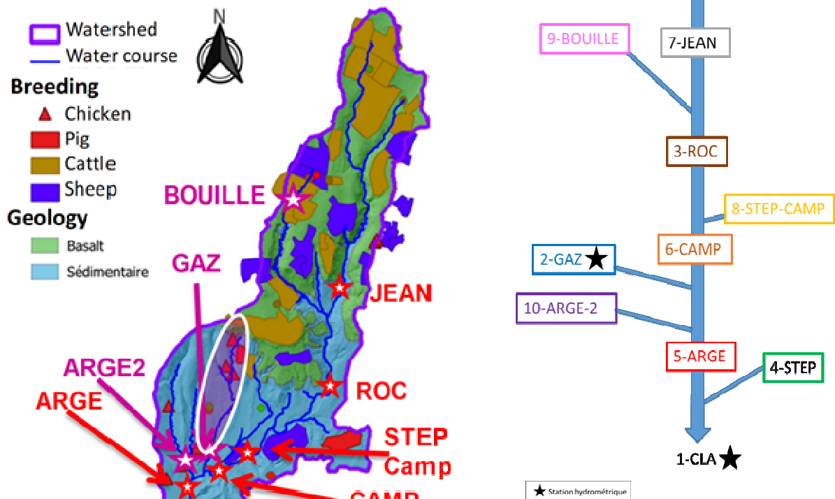
Figure 1 : Localisation des sites de prélèvement d'eaux de surface sur le site d'étude de la Claduègne (Ardèche). Les échantillons ont été respectivement prélevés (étoiles) soit directement dans le cours d'eau de la Claduègne (JEAN, ROC, CAMP, ARGE), soit dans des affluents (BOUILLE, STEP-CAMP, GAZ, ARGE-2, STEP)
