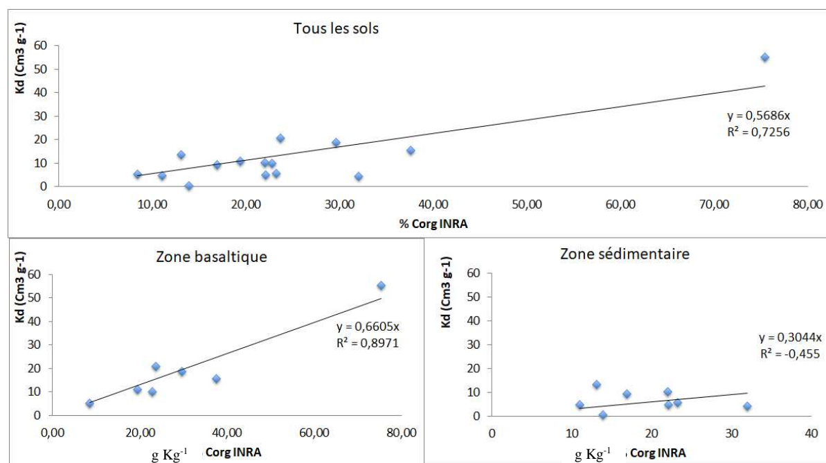
Figure 14 : Corrélation entre le K_d du SMX et la teneur en C_{\text{org}} de tous les sols (Haut) du bassin versant de la Claduègne (Ardèche), ou seulement des sols des zones basaltique ou sédimentaire (Bas).
