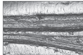
Fig. 5. Pointe expérimentale sur demi-métapode de chevreuil utilisée pour teiller des fibres de lin (grossissement \times 200 , © Y. Maigrot).
