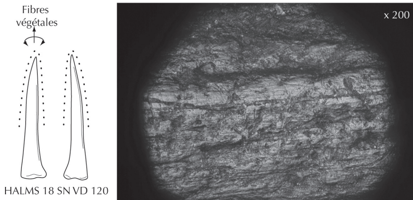
Fig. 6. Usure d'une pointe sur fibula de suidé interprétée comme le résultat du travail des fibres végétales (© Yolaine Maigrot).
