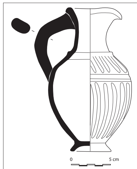
Figure 3 : Pichet à pâte calcaire et à décor de godrons incisés, Kellia, type 227, EGLOFF 1977, pl. 72, 2
