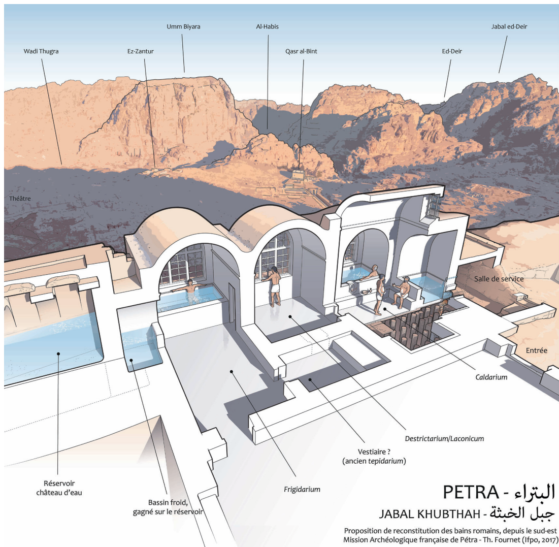
Fig. 6 : Proposition de restitution (perspective ouverte) des bains du Jabal Khubthah, depuis le sud-est (Th. Fournet, MAFP 2017)
