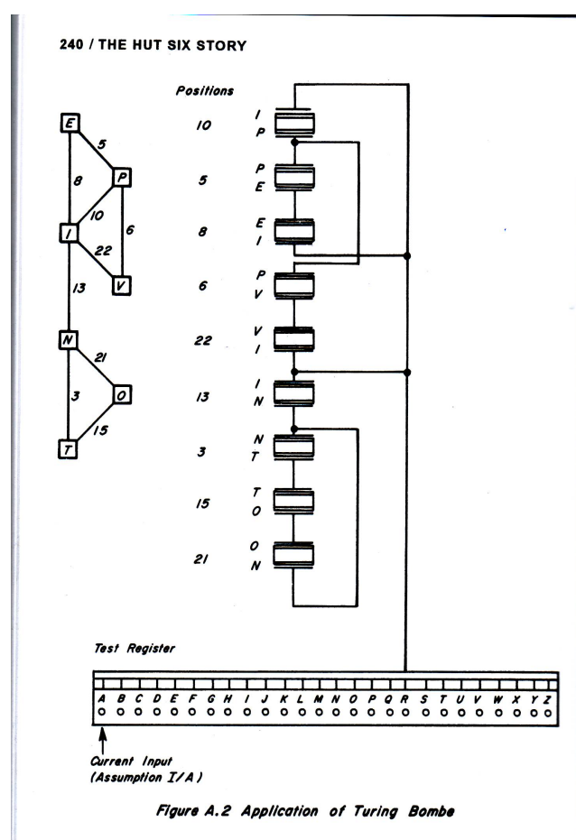
Fig. 7. Un menu et le montage associé de la Bombe (Welchman, 1982 [2017], p. 240) Avec l'autorisation des éditeurs M. & M. Baldwin
