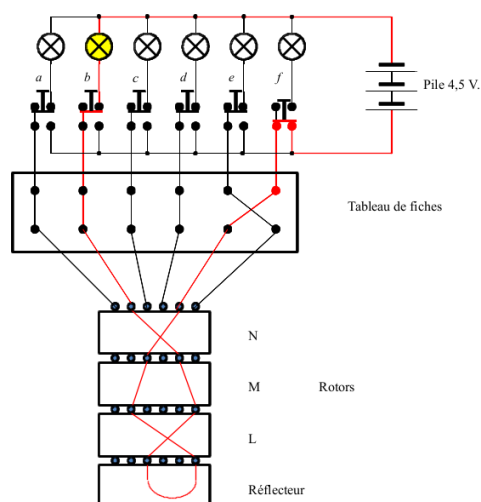
Fig. 2. Diagramme du chemin de chiffrement d'une lettre sur Enigma . Production des auteurs
