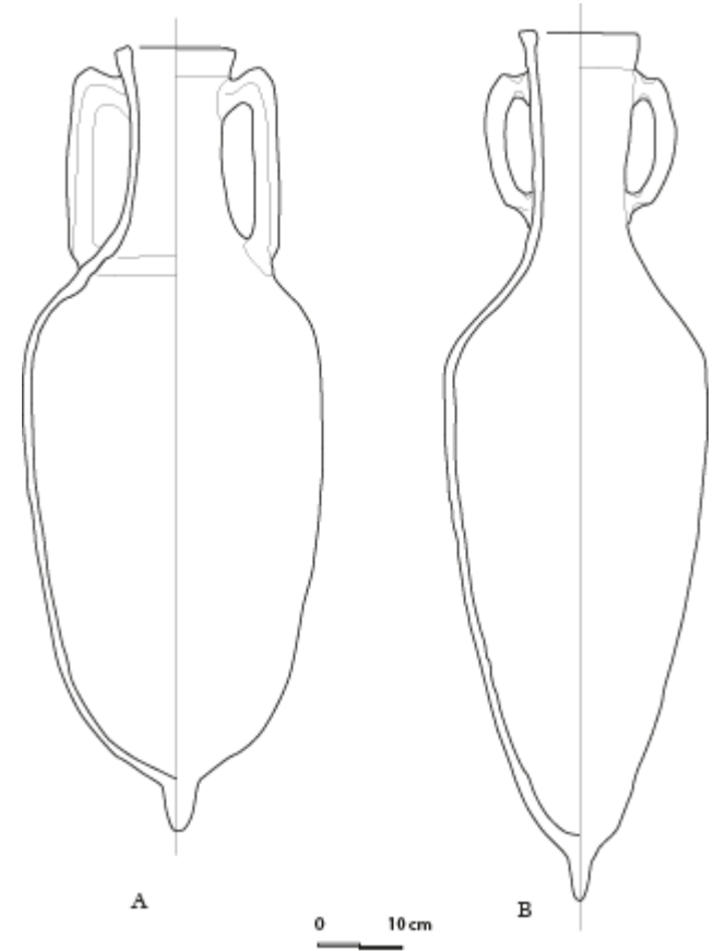
Amphores AE 2 produites à Tell el-Haraby (Majcherek, Shennawi 1991)
