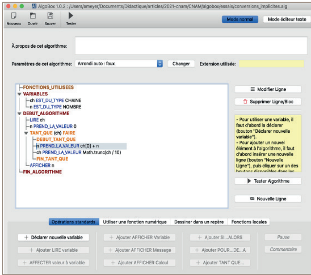
Figure 1 - Fenêtre principale d'AlgoBox (mode classique)
