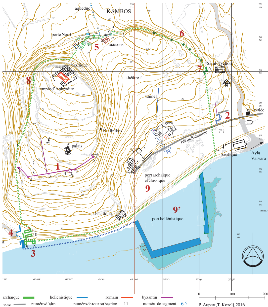
Fig. 1 — Plan simplifié des différentes phases de l'enceinte d'Amathonte. Relevé : M. et T. Kozelj; DAO : P. Aupert.
