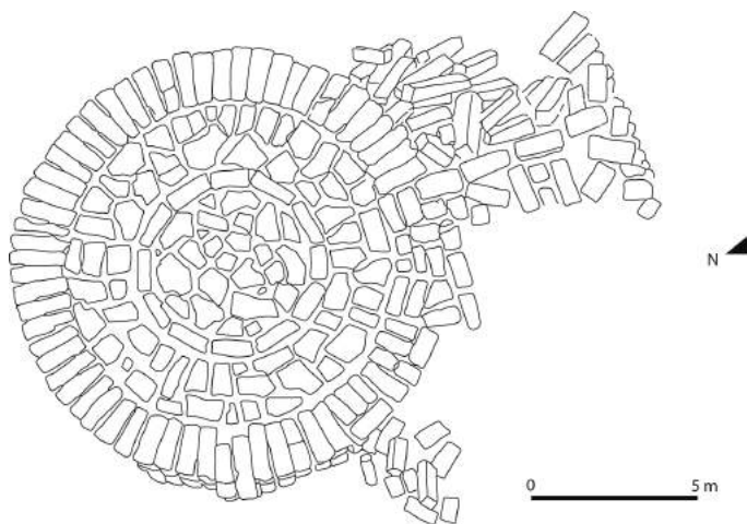
Fig. 3 — Plan de la tour à boutisses dans le port de la Tour de Straton (Césarée Maritime). Dessin E. Rossignol, in BALANDIER 2014b, p. 264, fig. 31.
