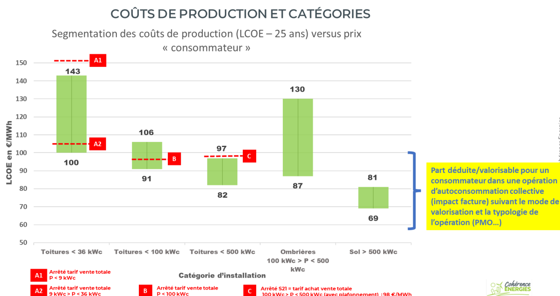
Figure 73 : Coût de production « photovoltaïque versus tarifs achat vente totale et « valorisation ACC » - Source : ADEME/Cohérence Energies
