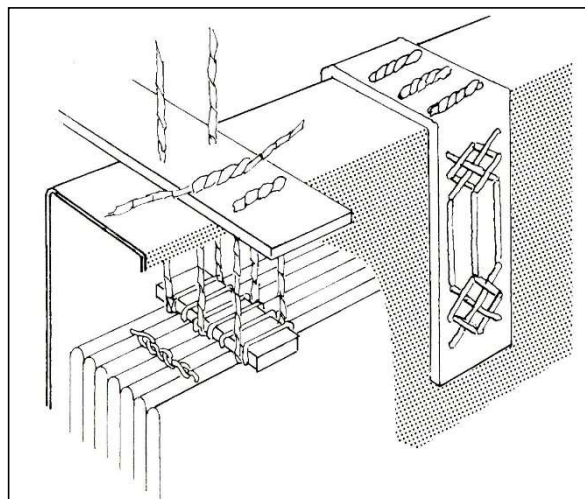
Ligature sur pattes de renfort
