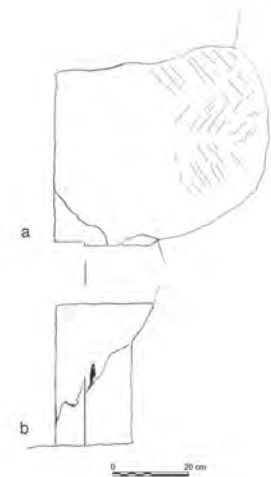
Fig. 11: Extrémité nord de la courtine hellénistique RMP1119. Bloc Us 2146 vu de haut (a) et face ouest (b). Relevé au 1:20e (dessin P. Fontaine)
