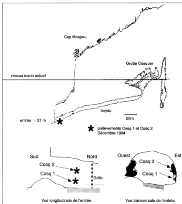
Fig. 2 : profil transversal de la grotte Cosquer et du couloir d'accès et de son entrée avec la position des prélèvements Mesophyllum lichenoides pour datation au radiocarbone. Source : Sartoretto et. al. , 1995
