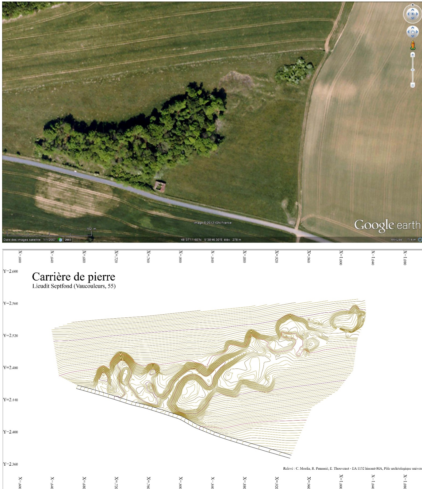
Fig. 6 – Carrière de calcaire de Meuse au lieudit Septfonds (Meuse). Vue satellite et relevé topographique (C. Moulis).
