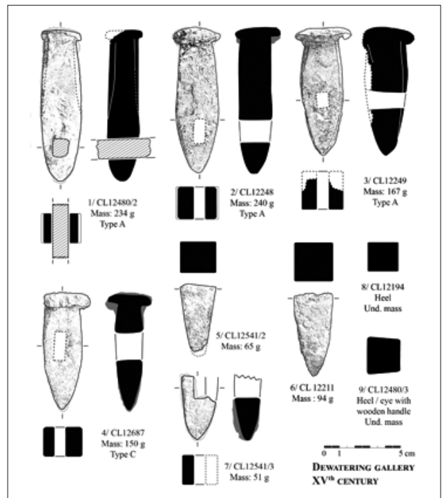
Fig. 10. Les Ouels, chisels from the dewatering gallery, 15th century. Obr. 10. Les Ouels, dláta z odvodňovací štoly, 15. století.
