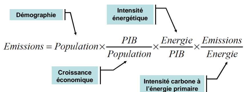
Figure 5. L'équation de Kaya D'après (GIEC, 2007 ; Crassous, 2008).
