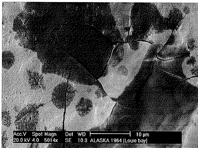
a) Vancouver 1964 SG : Aire de dislocation et réseau de fractures affectant un quartz non usé évolué
