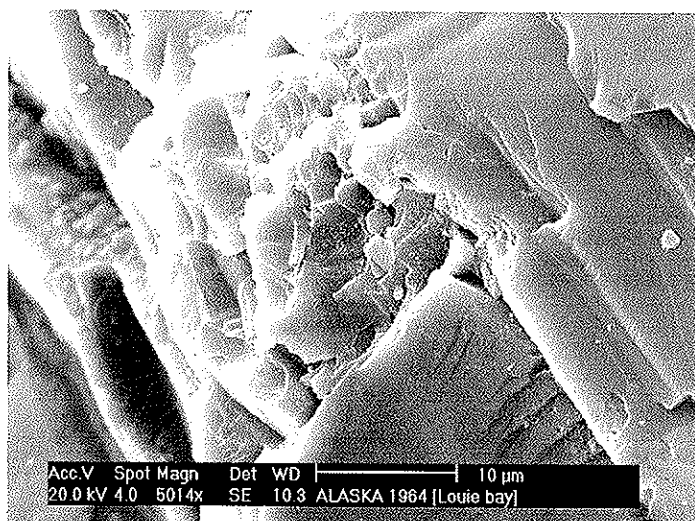
d) Vancouver 1964 SG : Secteur d'impact frais avec zone de broyage et écaillage important
