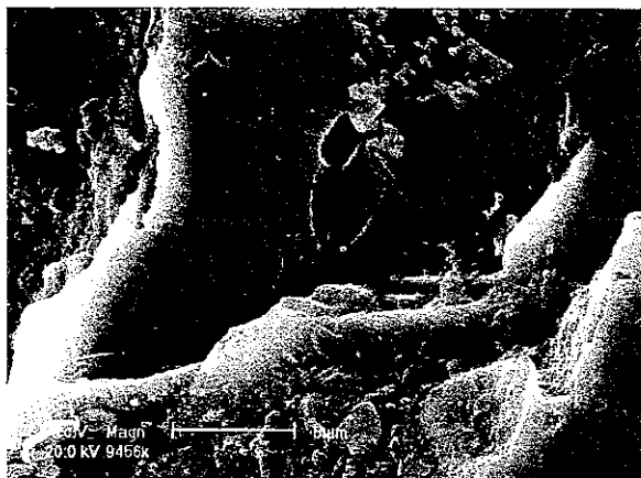
Photo 9 : Tsunami de 1755, quartz EL, sable moyen outre les quelques cupules de choc et les figures de microfracturation, présence de nombreuses écailles liées à la "desquamation", écailles qui se sont déposées et soudées (recristallisation car précipitation de la silice)
