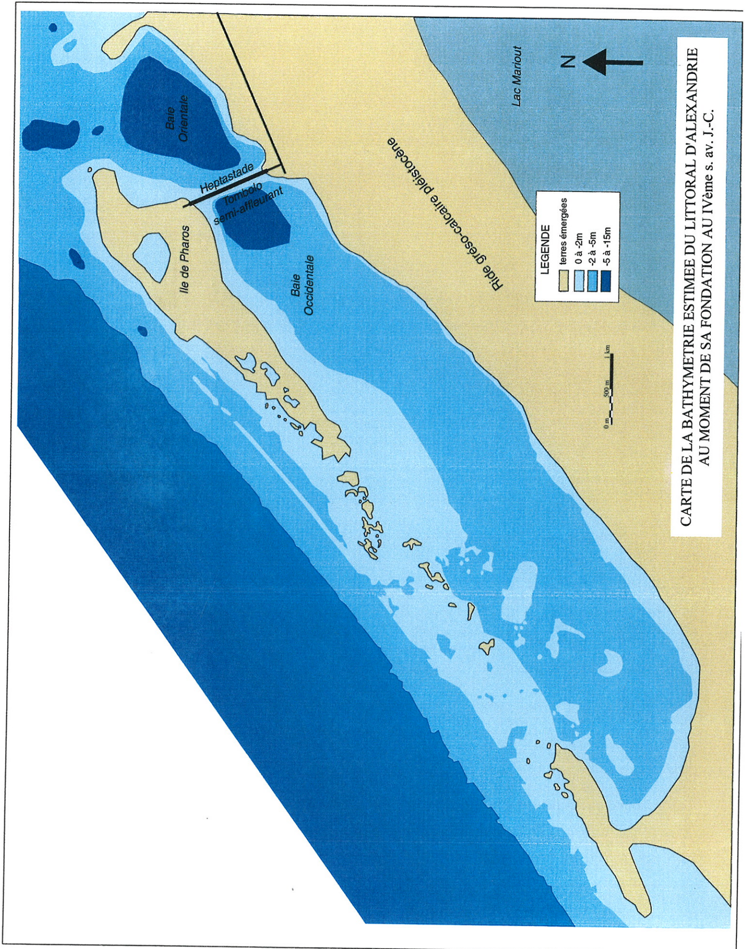
Figure 36 : Carte de la bathymétrie antique estimée
