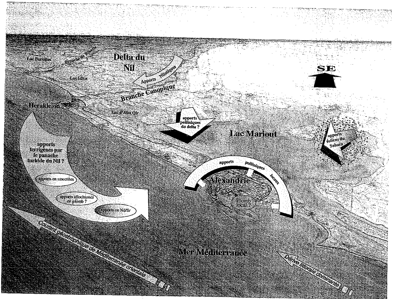
Figure 82 : Organisation des dynamiques et sources sédimentaires
