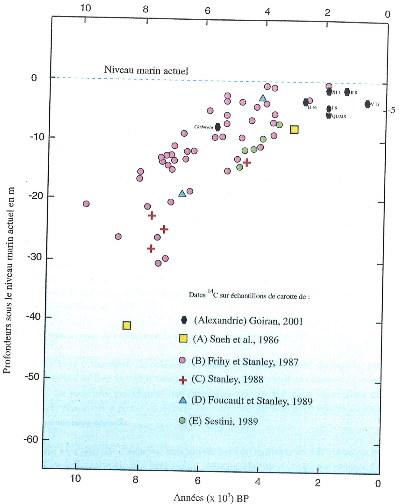
Figure 79 : Variations relatives du niveau marin holocène, sur plusieurs sites du delta du Nil.
