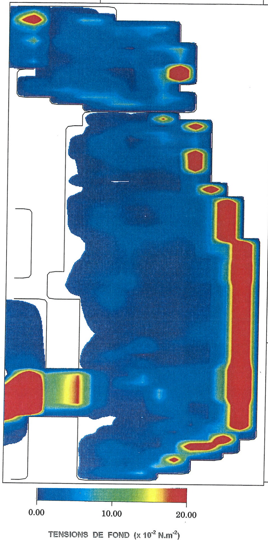
Figure 44 : Carte des tensions de fond résultantes (vague et courant) : situation après l'Heptastade
