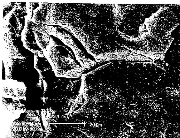
Photo 12 : Tsunami de 1755 quartz EL, sable moyen, microfracturation et zone de décollement
