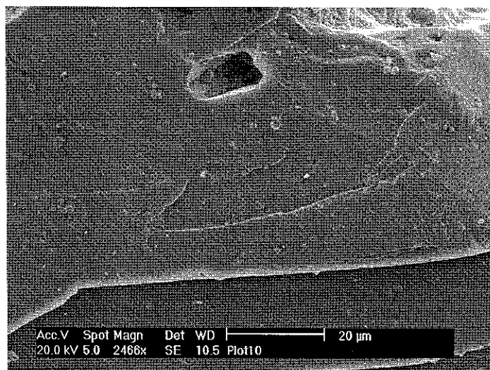
d) Alexandrie I 26 SM : Creux net sur une face, lié à une inclusion
