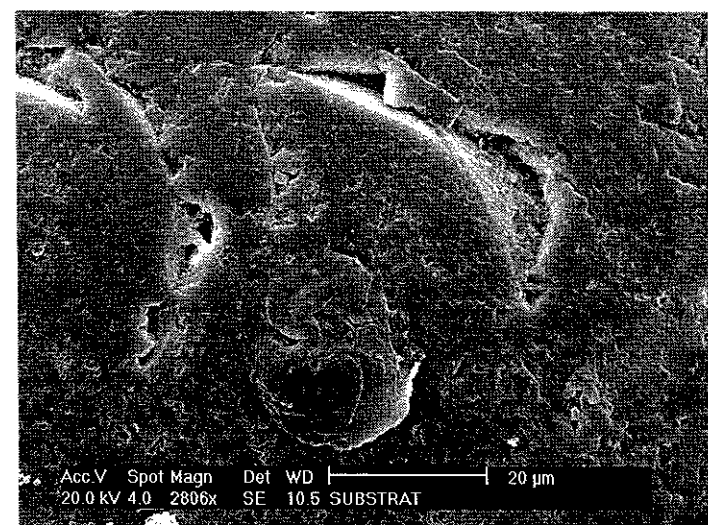
f) Alexandrie Substrat : Cupules de chocs
