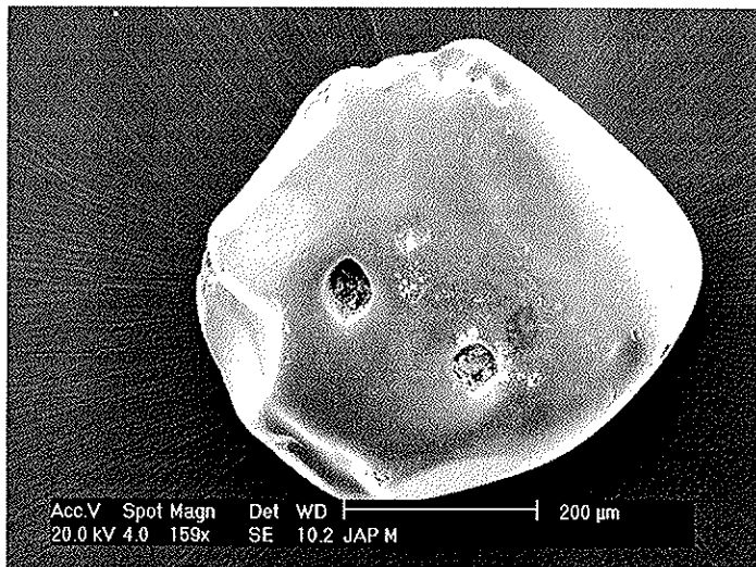
a) Japon 869 SM : Quartz émoussé luisant avec inclusions
