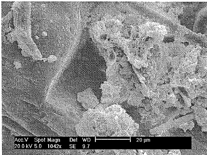
c) Alexandrie I 17 SM : Alvéole d'inclusion remplie de dépôts, fragments de diatomées et de baguettes de gypse
