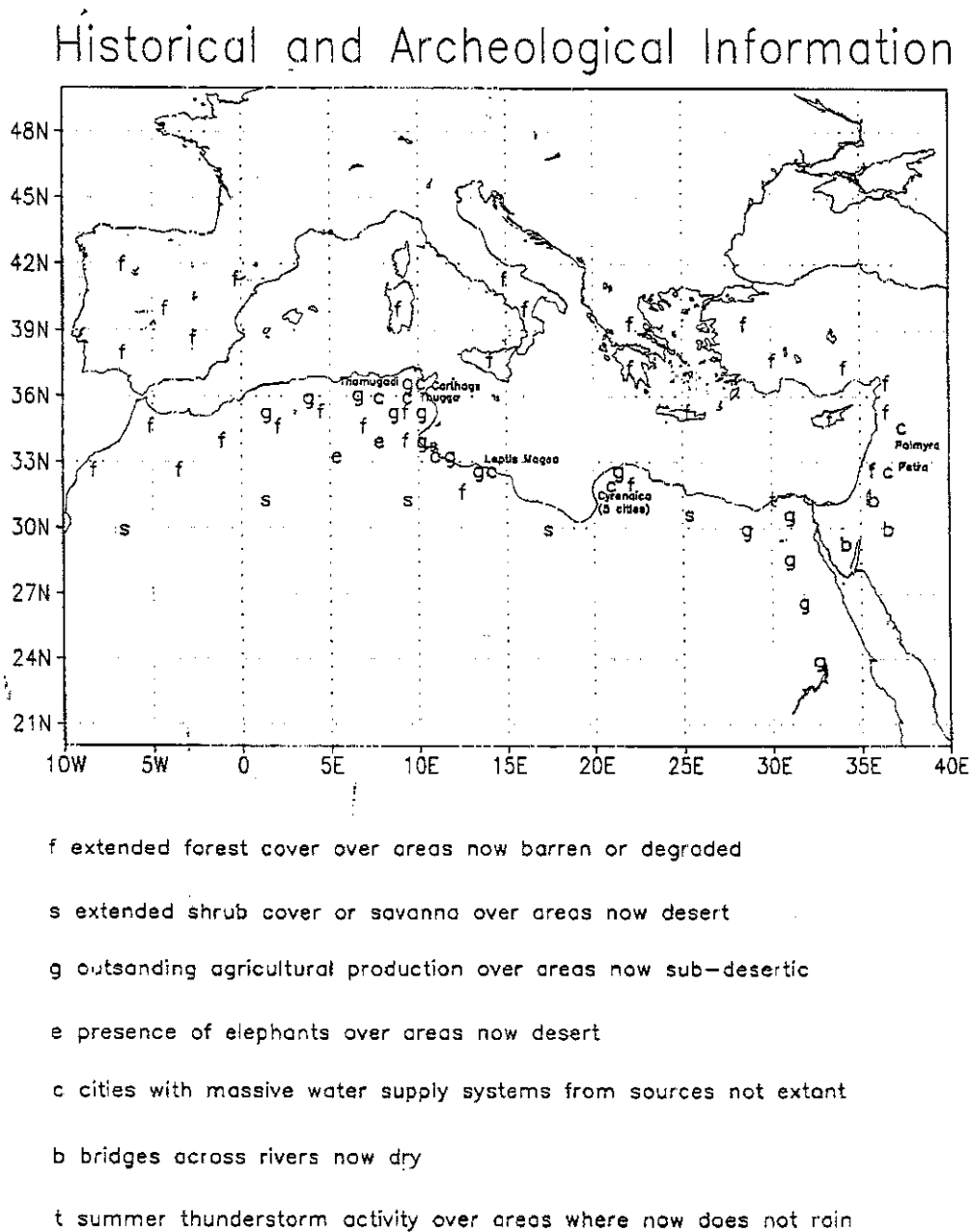
Figure 96 : Carte qualitative des changements climatiques et/ou paysagers déduite des sources littéraires et des données archéologiques (source : Reale et Dirmeyer P., 2000)
