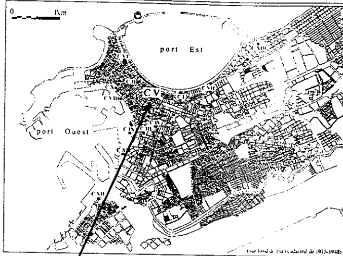
Figure 52 : Localisation du carottage C V : Khan Chorbagy
