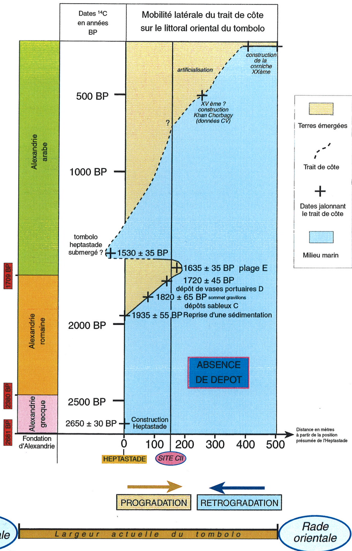
Figure 32 : Mobilité latérale du trait de côte sur le tombolo d'Alexandrie à partir des données de la carotte II
