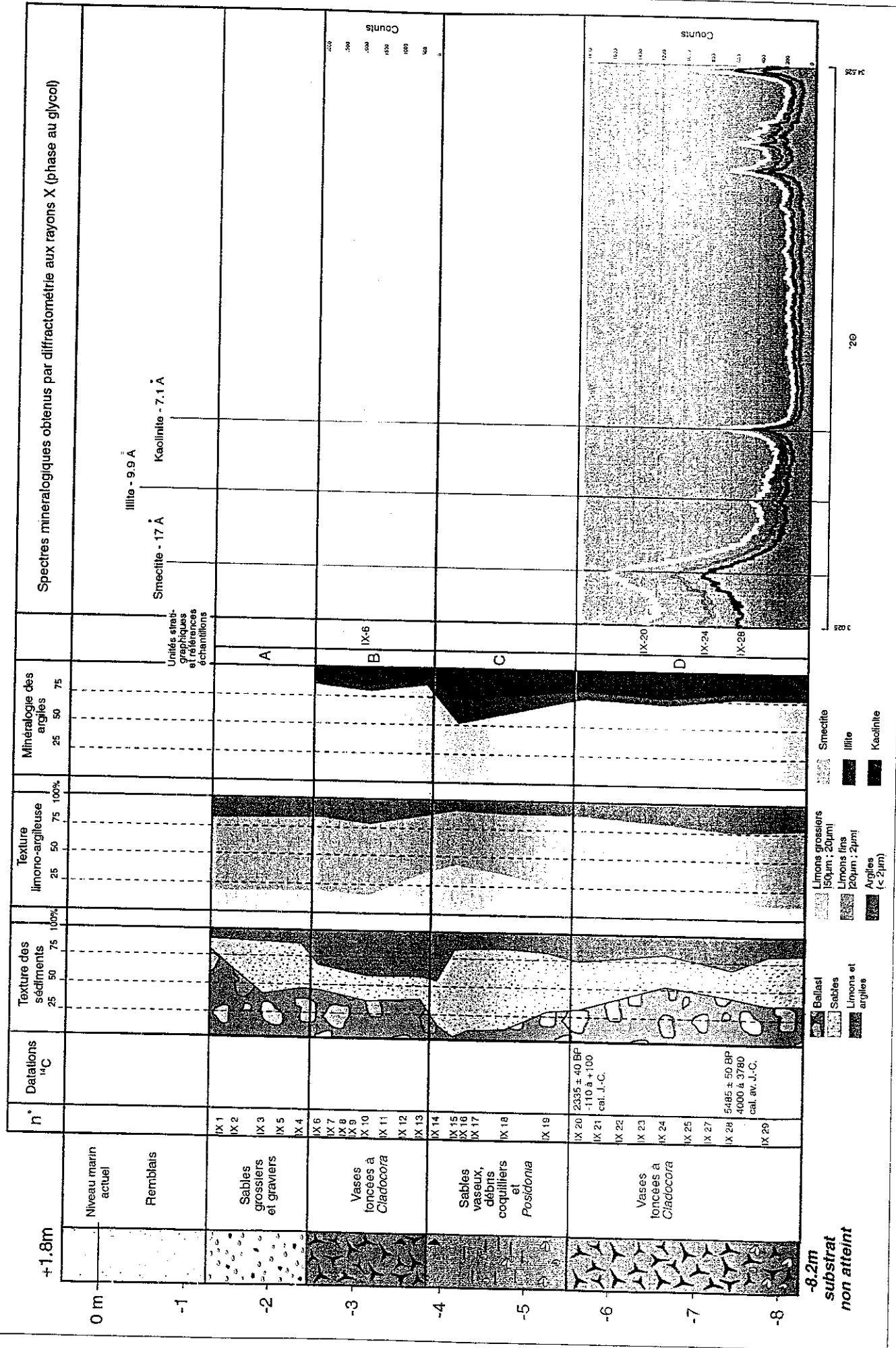
Figure 83 : Minéralogie de la phase argileuse : carotte C IX Bureau des Douanes
