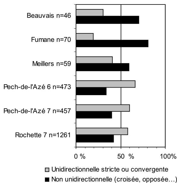
Histogramme VI 4. Direction des enlèvements d'après les éclats dans des industries discoïdes (déduites des illustrations de Loch et Swinnen, 1993; Loch et al., 1995 ; Peresani, 1998 ; Pasty, 2000 respectivement) et dans les industries à éclats allongés étudiées
