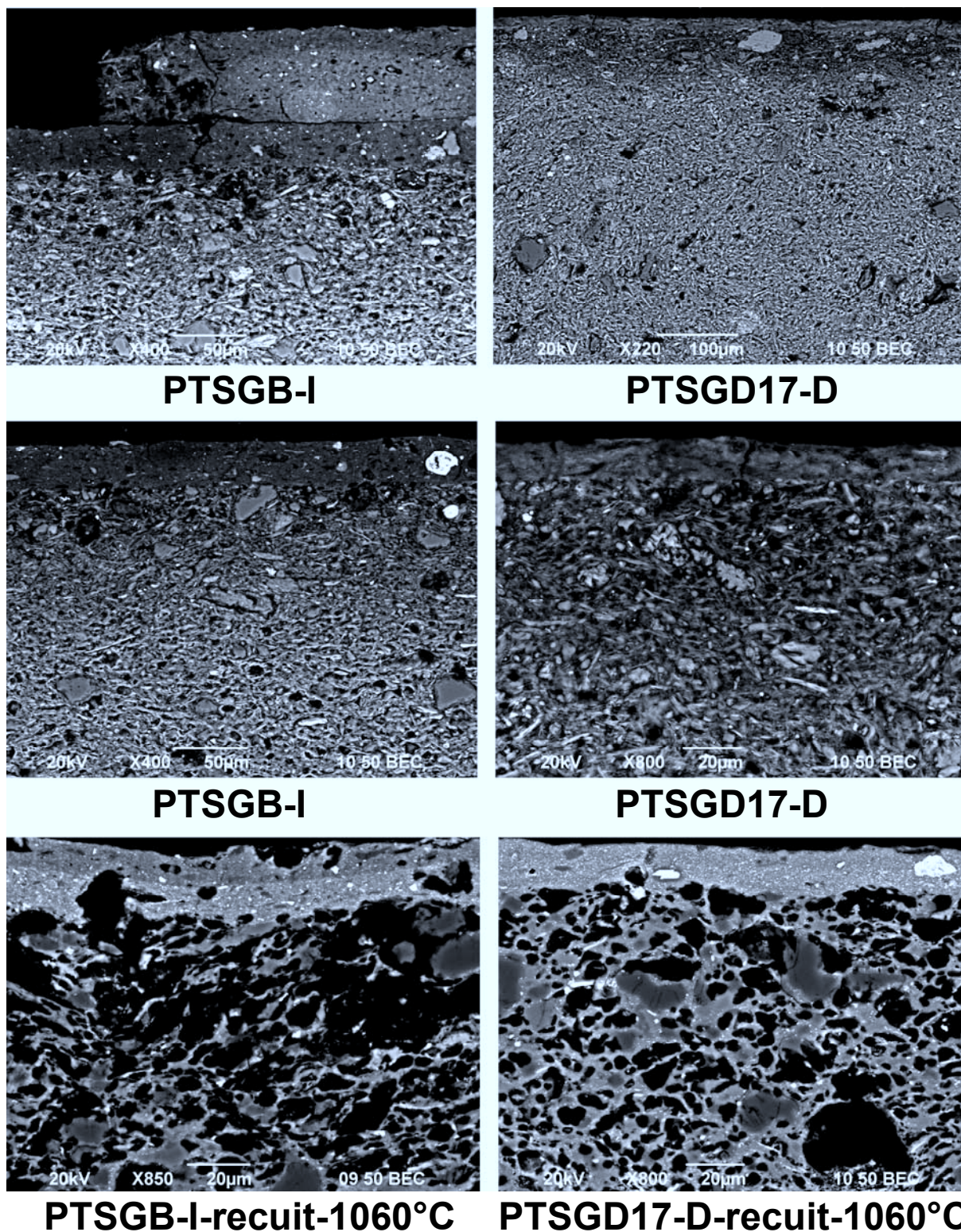
Figure V.C.3 : Coupes transverses polies de fragments de sigillées à engobe siliceuse non vitrifié rouge et noir riche en fer, provenant des ateliers de La Graufesenque, observées par MEB en mode électrons rétrodiffusés.
