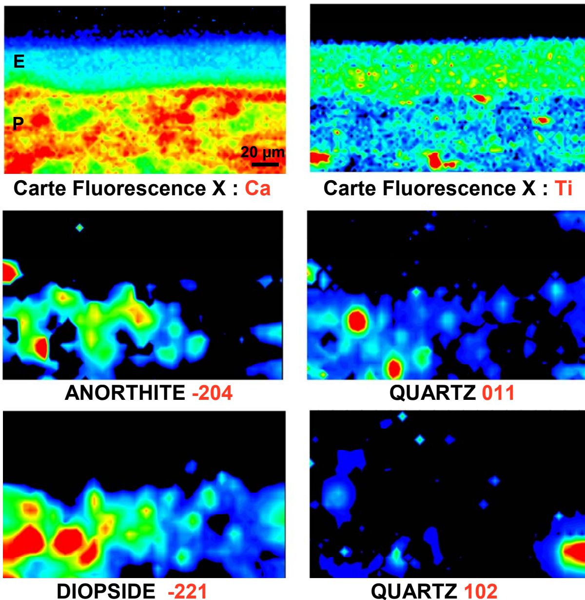
Figure III.D.17 : Cartographies \mu XRF (pas = 2 \times 2 \mu\text{m}^2 ) du calcium et du titane, et cartographies minéralogiques associées (pas 4 \times 4 \mu\text{m}^2 ) de l'anorthite, du diopside et du quartz obtenues en intégrant l'intensité d'un anneau de diffraction, réalisées sur la coupe du fragment TSMFEL1 attribué à l'atelier de Montans. La couleur rouge est associée aux concentrations maximales, la couleur bleu aux concentrations minimales et les zones noires correspondent à une concentration nulle.
