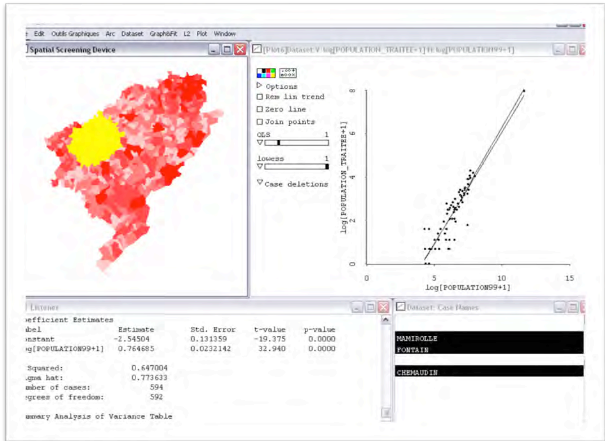
Figure 11 : L'interface GWR de GéoGrapheur. Le même modèle (ici une régression linéaire) est calculé localement, au sein de la fenêtre de sélection spatiale, les entités spatiales étant pondérées en fonction inverse de leur distance au centre de la fenêtre (GéoGrapheur).
