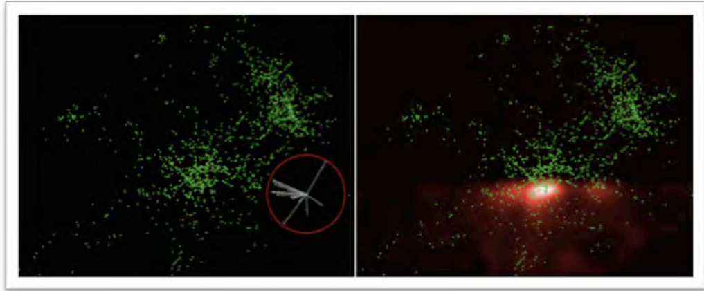
Figure 47: Le lissage par noyaux (Kernel Density Estimation) développé dans SMArtKDE. Une surface (densité de probabilité) est construite à partir du semis de points initial, grâce à une fenêtre mobile circulaire (kernel) parcourant la zone (SMArtKDE).
