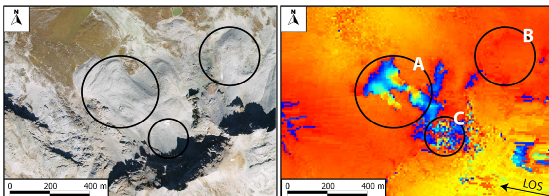
Figure 32 : Illustration des différents types d'informations utilisés sur les interférogrammes. Les lettres se réfèrent aux explications fournies dans le paragraphe précédent. Glacier rocheux nord-ouest de la pointe de la Vallaisonnay ; à gauche : ortho-image de 2006 ; à droite : interférogramme à 11 jours de la même zone provenant de données TerraSAR-X de 2013. LOS : Line Of Sight : ligne de visée du satellite (sur le plan horizontal).
