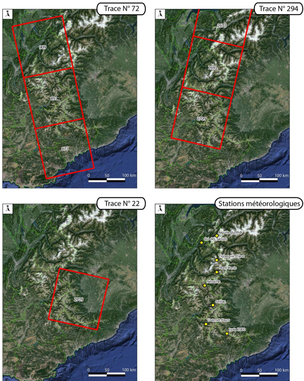
Figure 41 : Localisation des scènes d'archives ERS commandées et des stations météorologiques utilisées. Le numéro des traces figure dans le titre de chaque carte et les numéros des sections de trace (les scènes) figurent dans les carrés les délimitant. Sur la carte en bas à droite, les points jaunes localisent les stations météorologiques de MétéoFrance retenues pour les données de précipitations.
