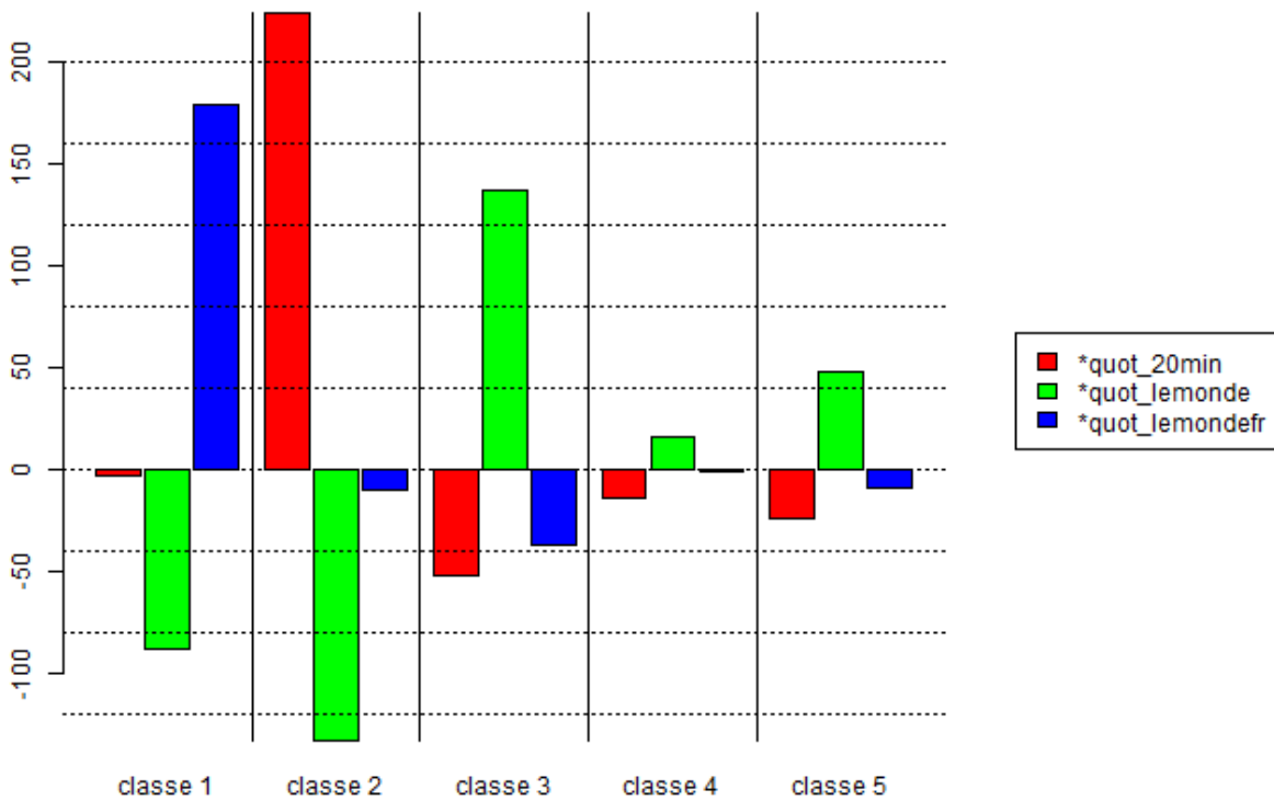
h. \chi^2 modalités de la variable « quotidien »
