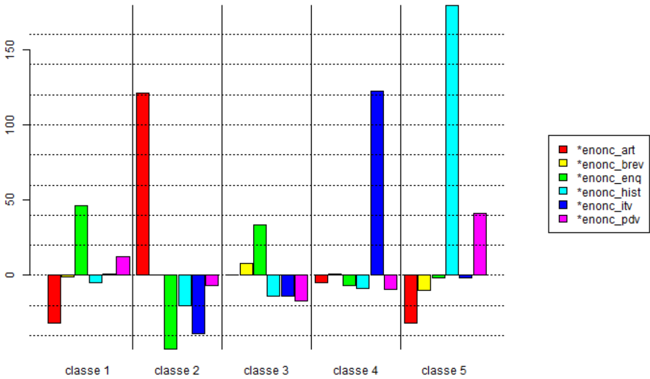
g. \chi^2 modalités de la variable « énonciation »
