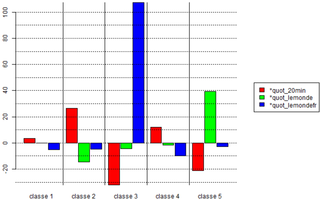
h. \chi^2 modalités de la variable « quotidien »
