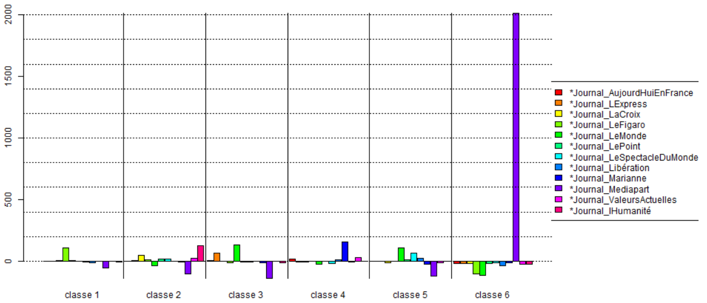
d. Khi2 modalités de la variable « journal »
