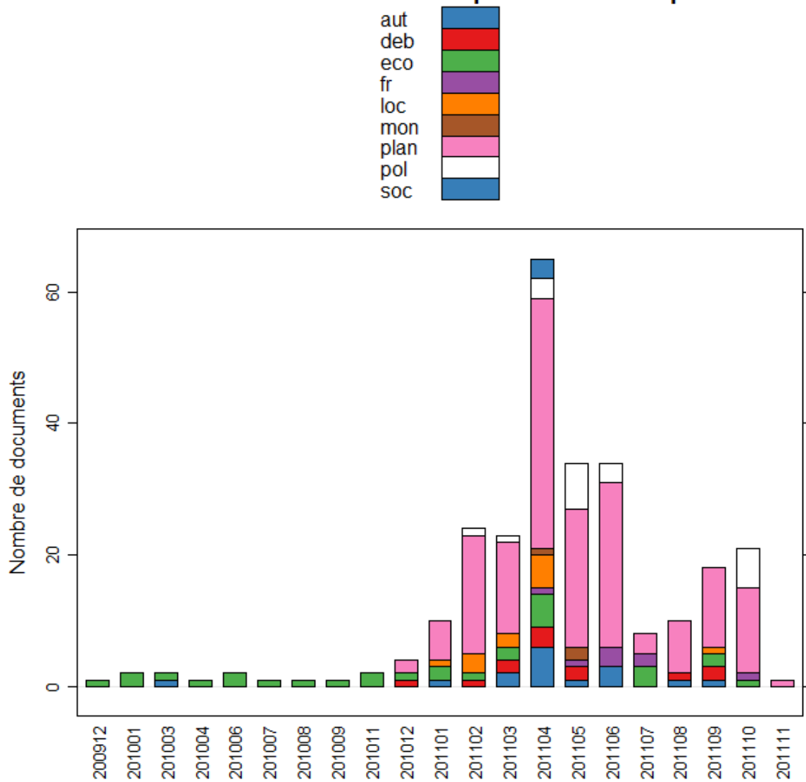
Distribution des documents par date et rubrique
