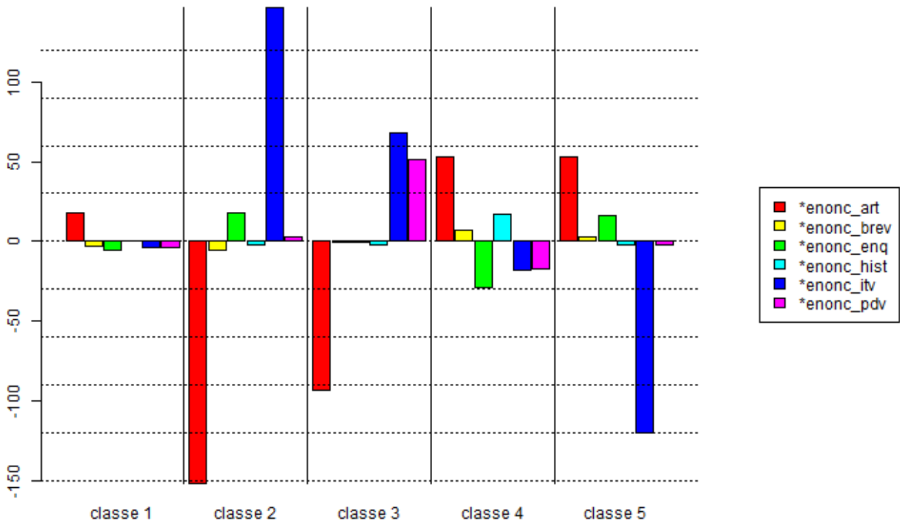
h. \chi^2 modalités de la variable « quotidien »
