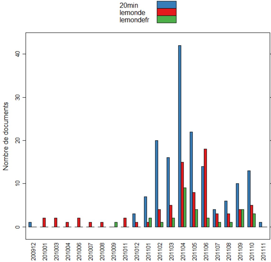
Distribution des documents par date et quotidien
