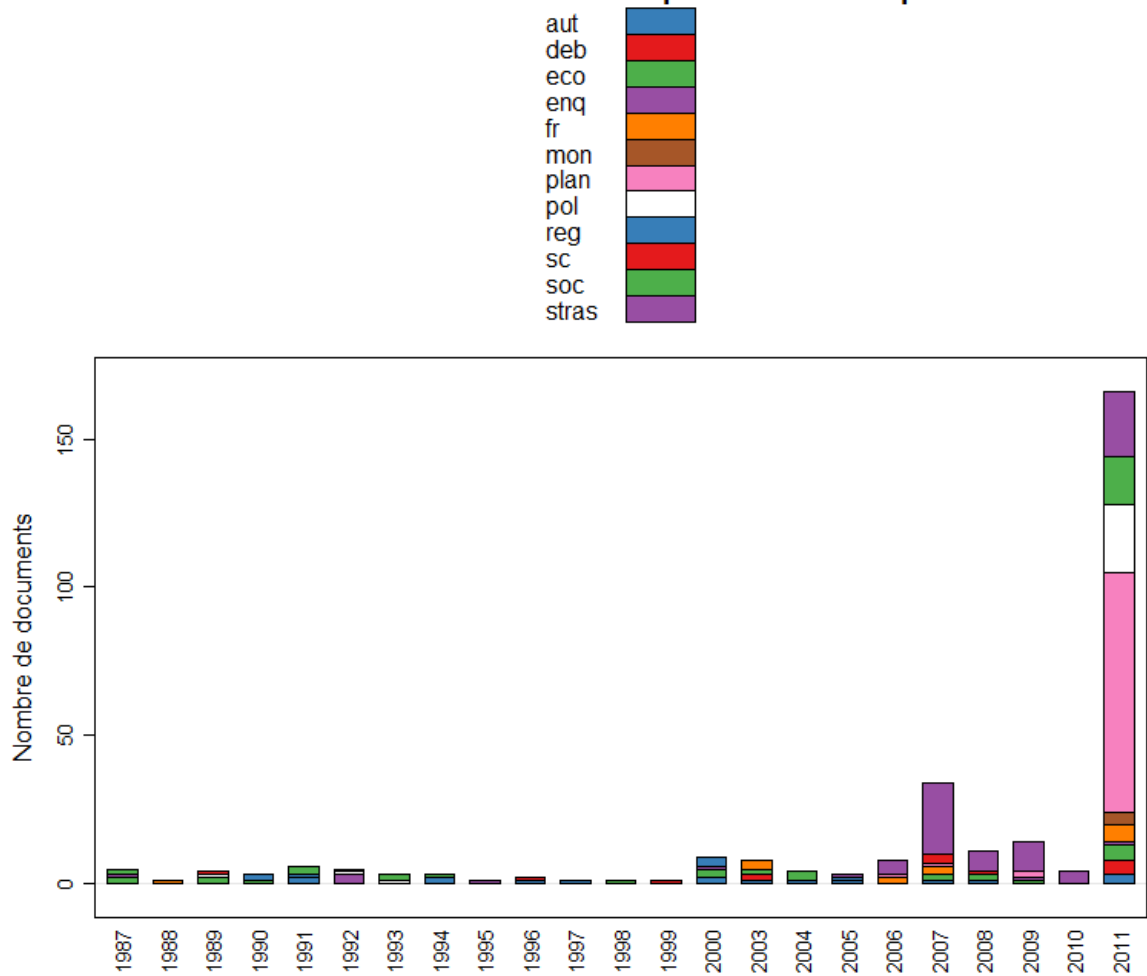
Distribution des documents par date et rubrique
