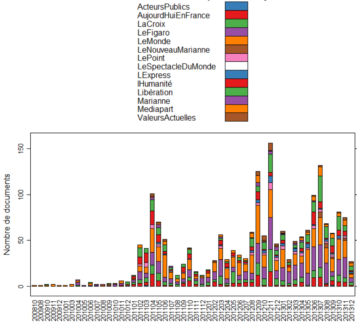
Distribution des documents par date2 et journal
