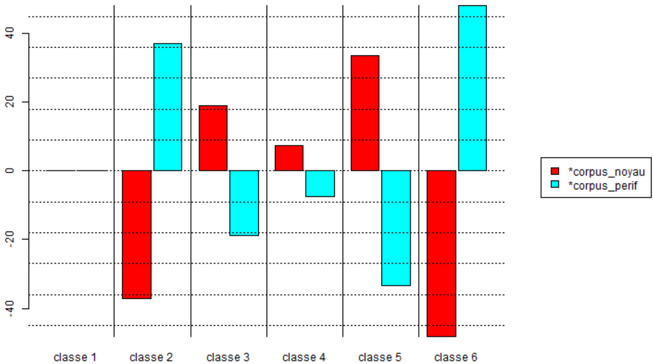
e. Khi2 modalités de la variable « corpus noyau / périphérique »
