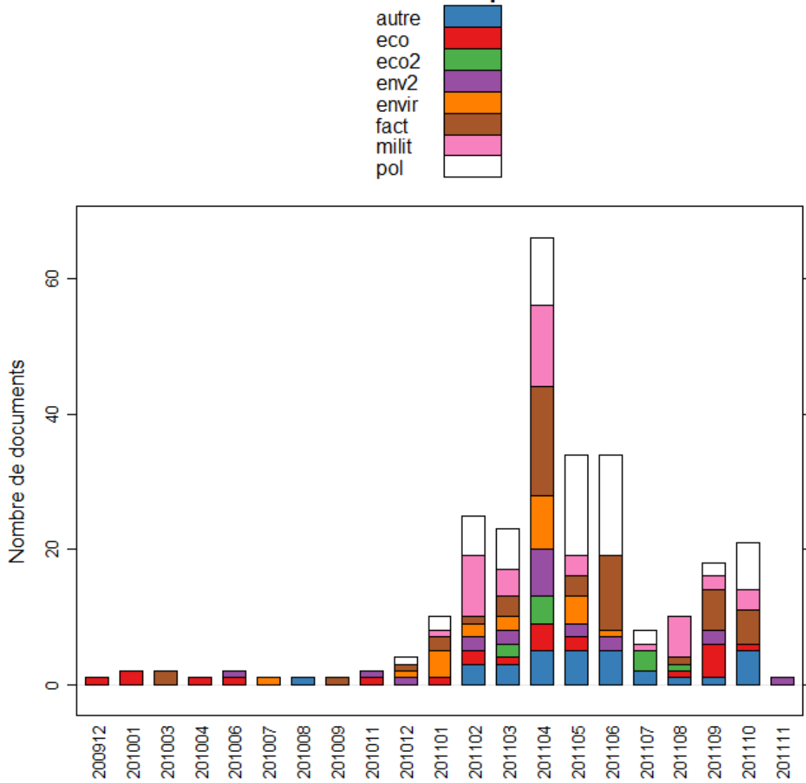
Distribution des documents par date et cadre
