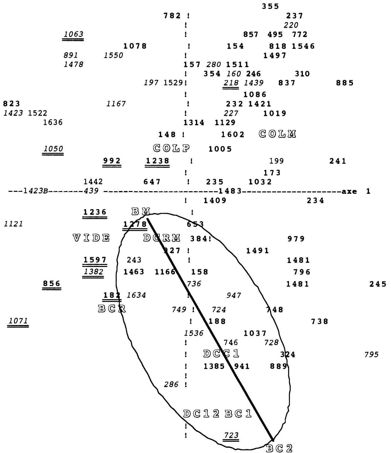
Fig.19. AFC 10 aucun point superposé
