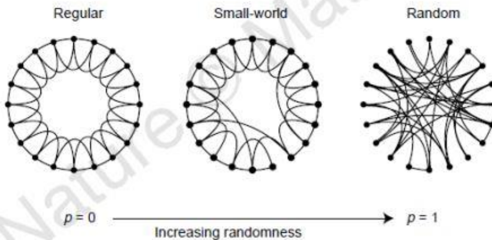
Figure 8 : Illustration des modèles de réseaux théoriques
