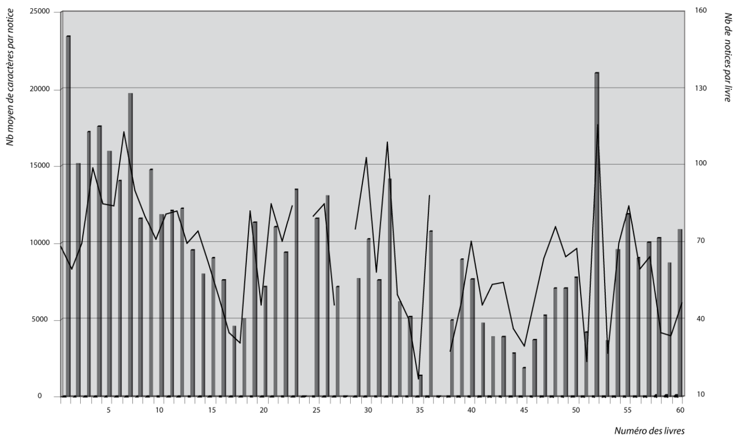
Fig. 6 – Nombre de caractères (histogramme) et de notices (courbe) par livre.
