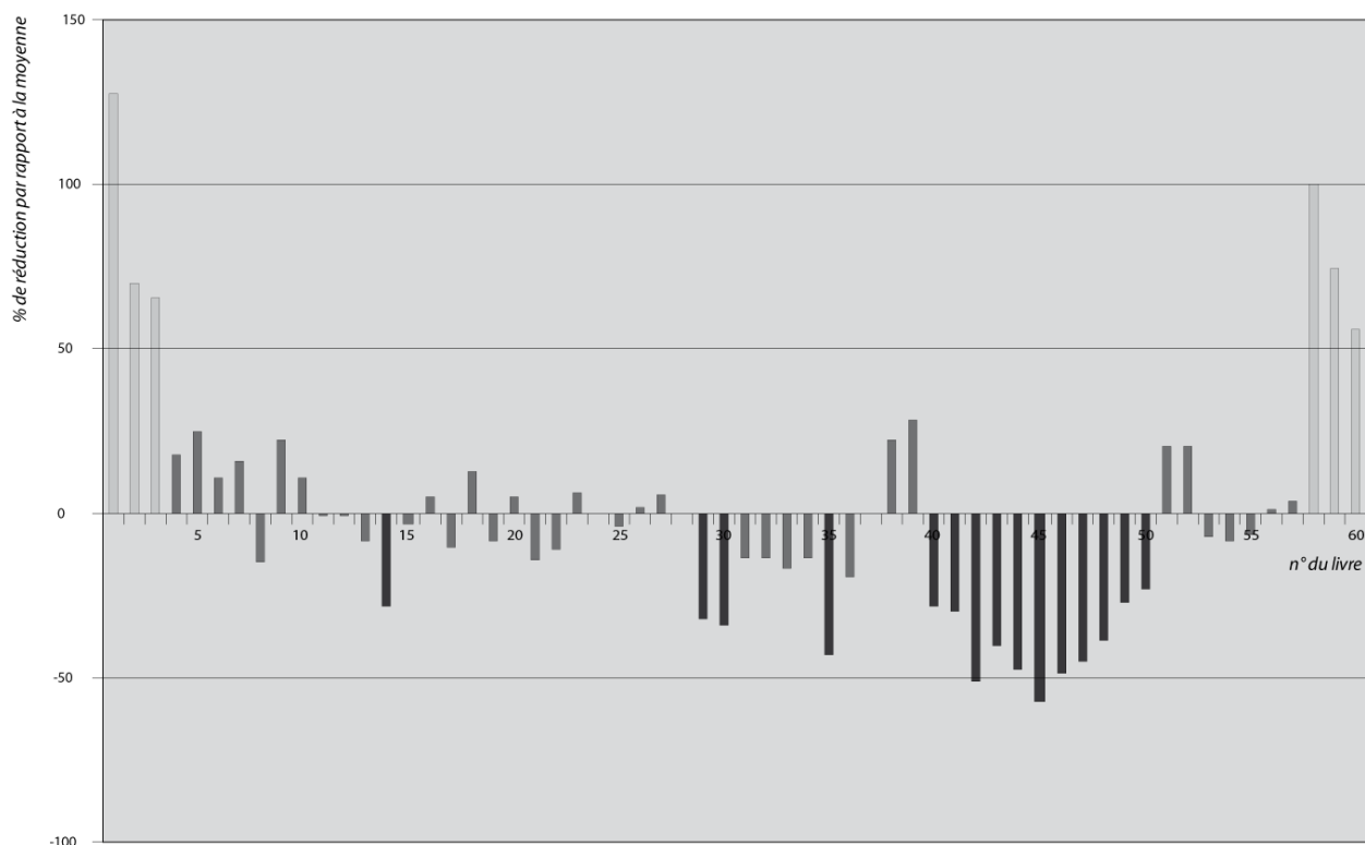
Fig. 7 – Pourcentage de réduction des 60 livres de Stéphane de Byzance par rapport à la moyenne.
