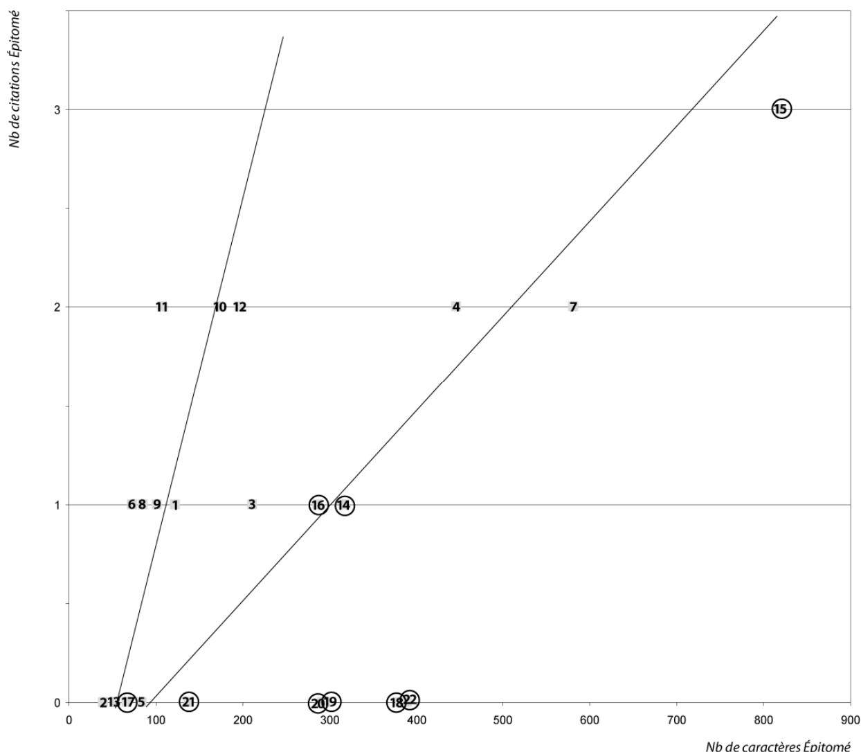
Fig. 4 - Rapport entre le nombre de caractères et le nombre de citations dans l'Épitomé.
