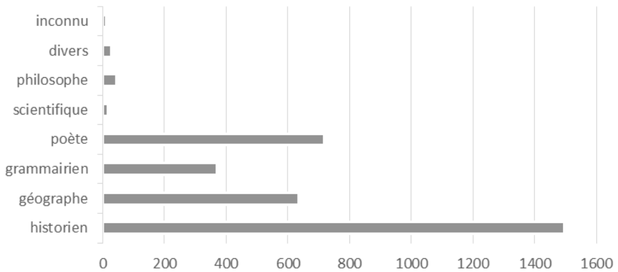
Fig. 13 – Répartition des types d’auteurs par nombre de mentions.
