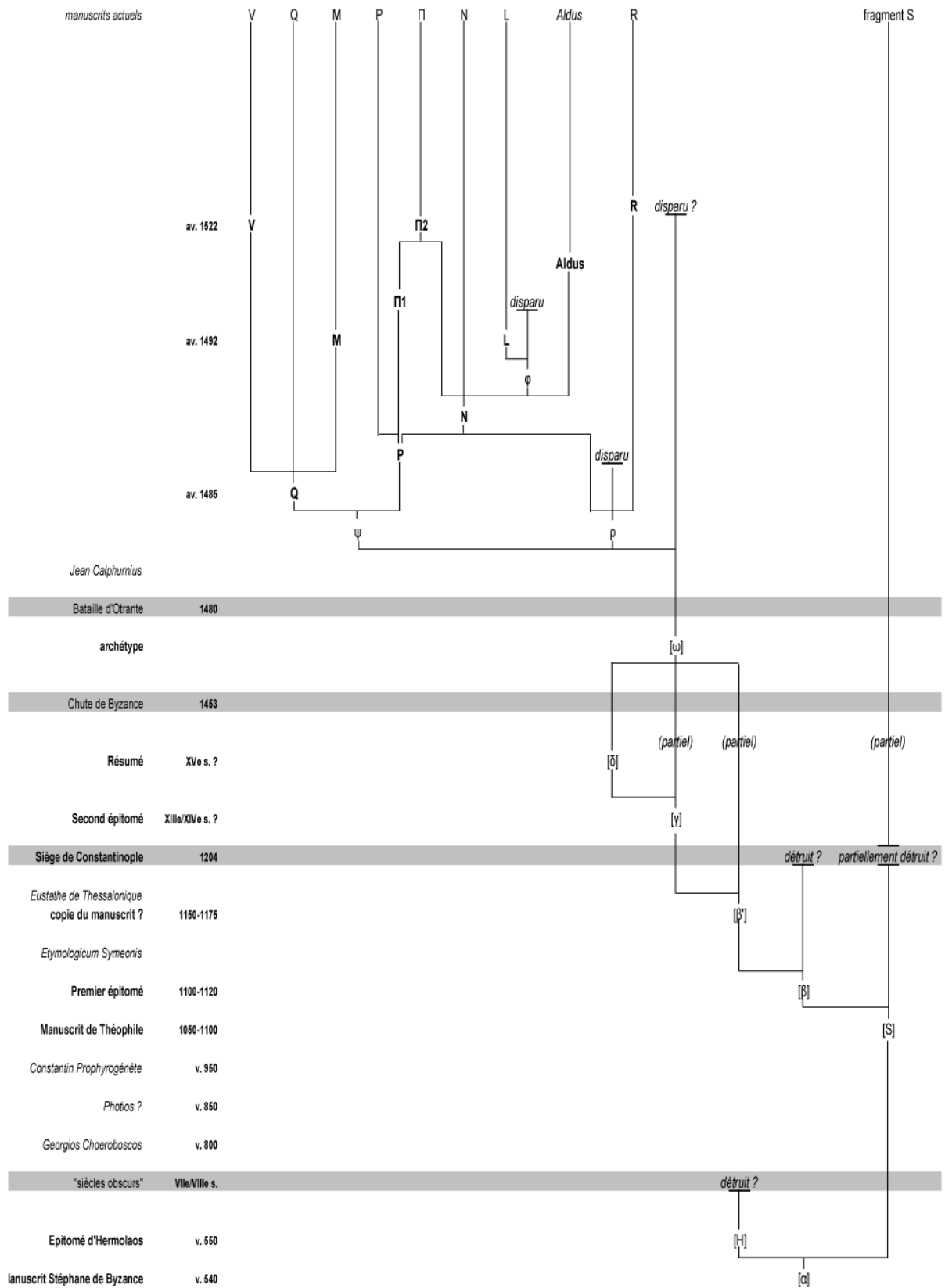
Fig. 10 – Diagramme chronologique de la tradition manuscrite (d'après Billerbeck 2006, p. 29* pour la partie haute).
