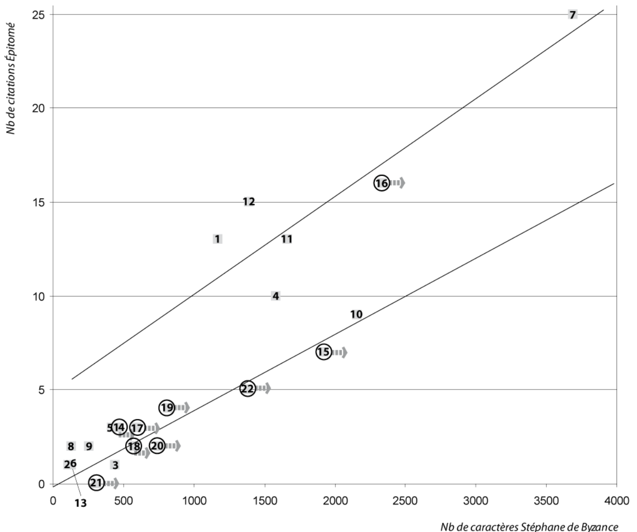
Fig. 3 - Rapport entre le nombre de caractères et le nombre de citations chez Stéphane de Byzance et droites de corrélation des deux groupes.
