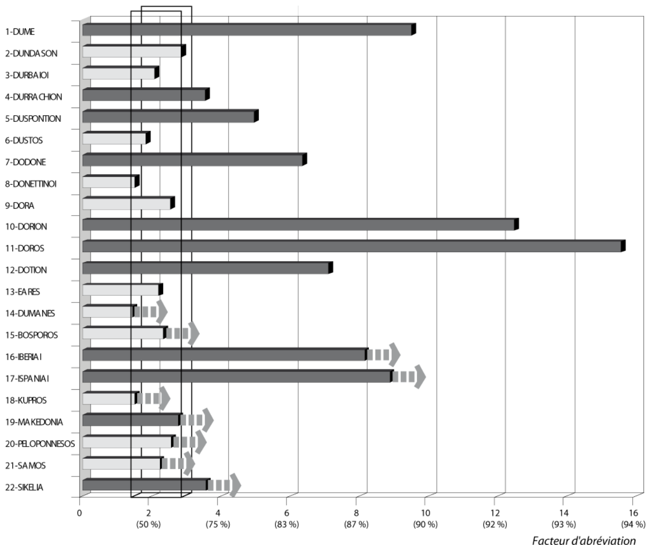
Fig. 2 – Facteur d’abréviation des notices.
