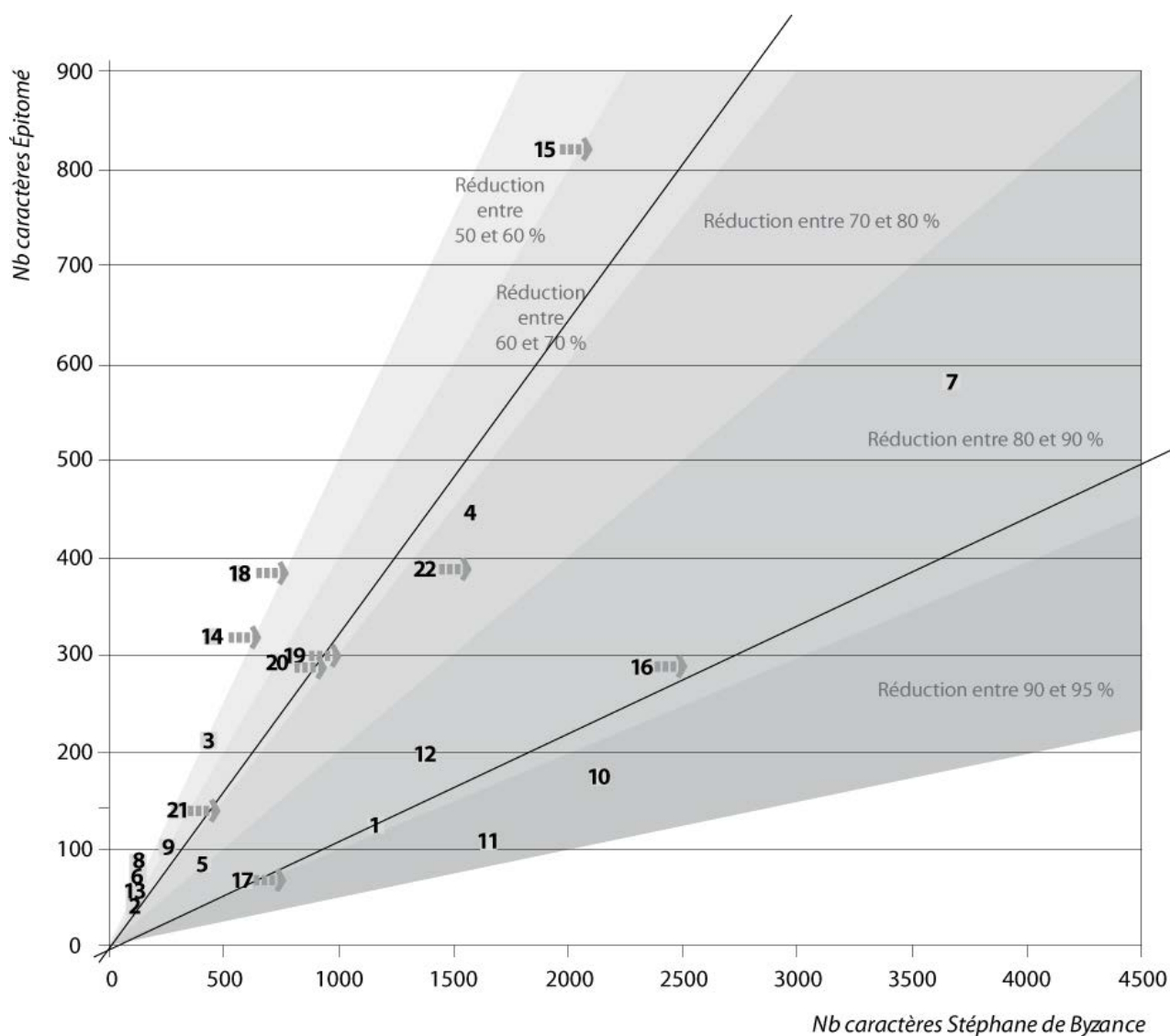
Fig. 1 - Rapport entre le nombre de caractères par notice chez Stéphane de Byzance et l'Épitomé et droites de corrélation des deux groupes.
