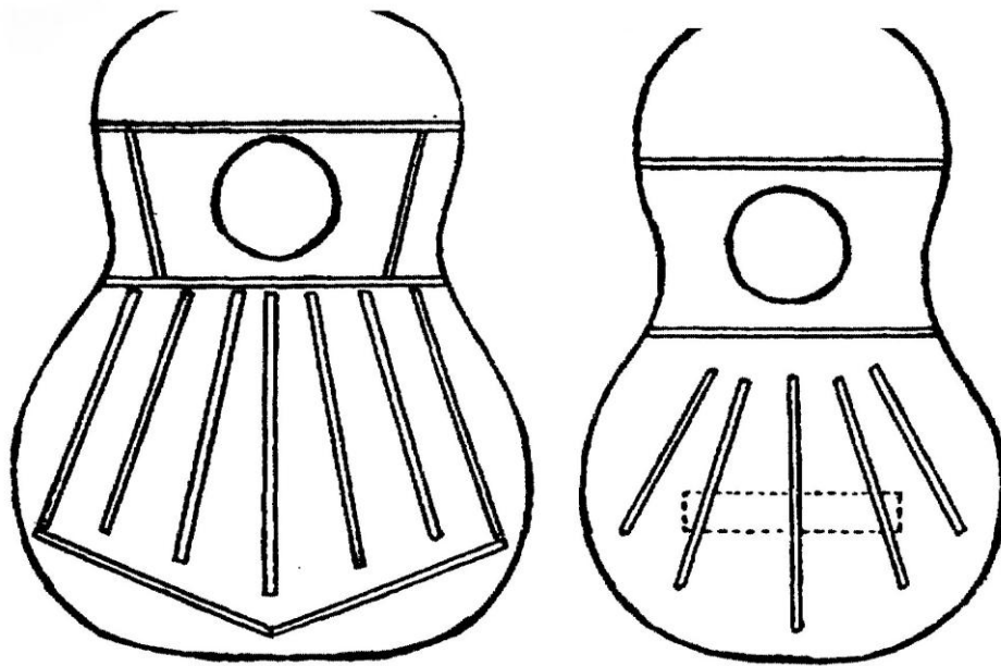
Figure 1 : barrage en éventail à sept branches (guitare classique) ou à cinq (flamenca) 541
