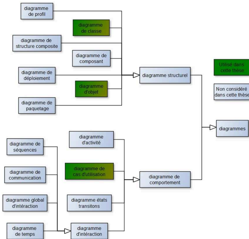
FIG. 3.5 – Arborescence des diagrammes en UML, d'après [Audibert, 2014].
